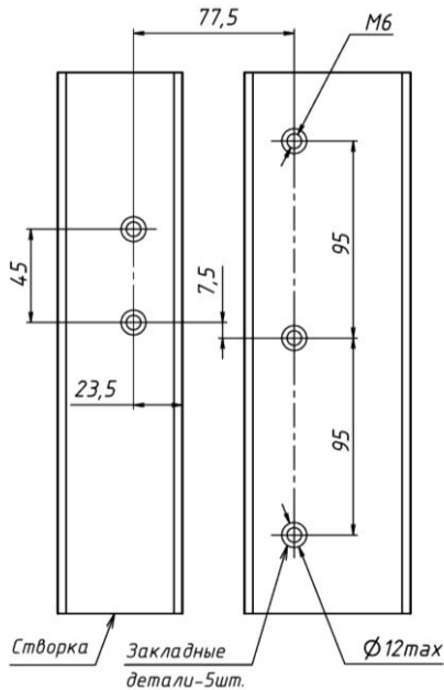
Рисунок 2 – Установка закладных деталей
