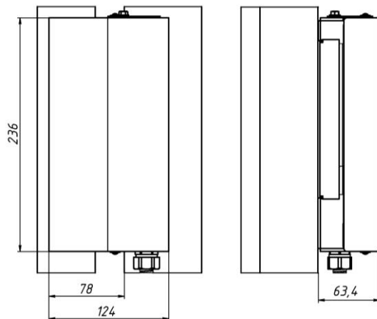
Рисунок 5 - Габариты комплекта в проеме двери
