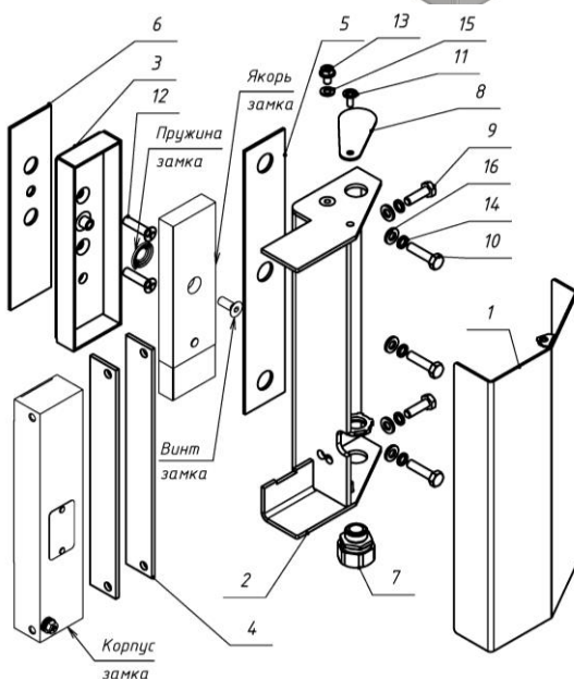
Рисунок 1 – Комплект МК FM-M22-GP
