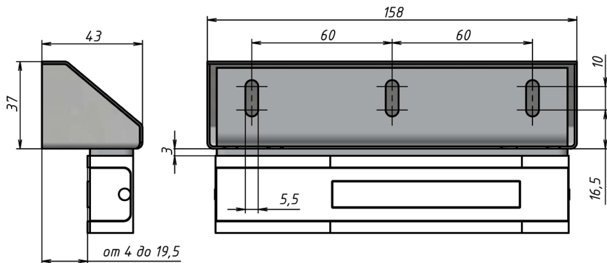
Рисунок 2 - Габаритный чертеж
