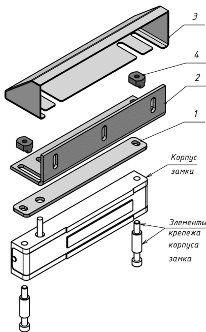
Рисунок 1 – Комплект поставки
