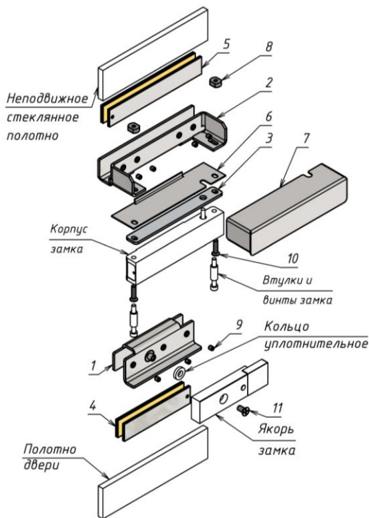
Рисунок 1 – Комплект поставки
