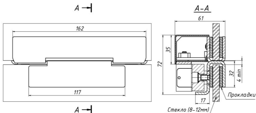
Рисунок 2 - Габаритный чертеж комплекта МК 150-GL
