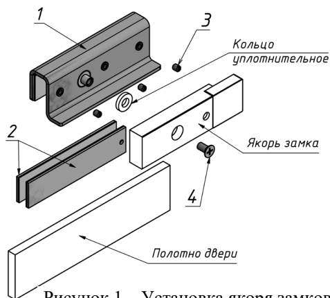
Рисунок 1 – Установка якоря замков ALM-150P и AL-150 PRemium
