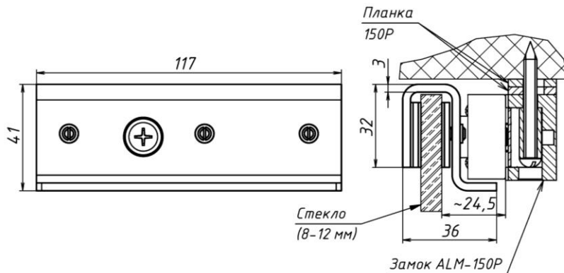
Рисунок 2 - Габаритный чертеж комплекта МК 150-GLU
