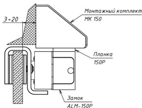
Рисунок 3 – Установка замка ALM-150P на стеклянную дверь с комплектами МК 150 и МК 150-GLU
