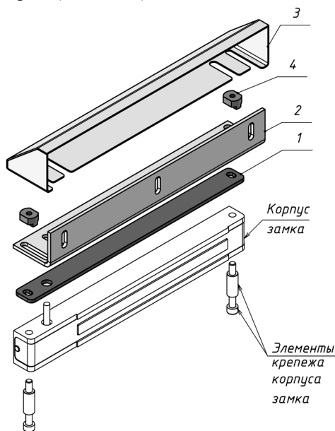
Рисунок 1 – Комплект поставки
