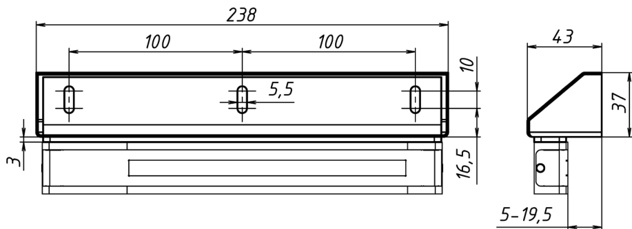
Рисунок 2 – Габаритный чертеж
