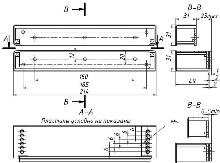
Рисунок 2 – Габаритно-установочные размеры комплекта МК 400S-PS
