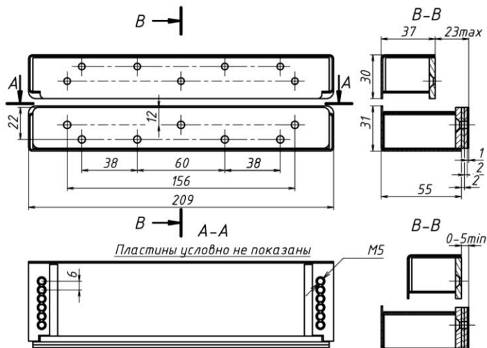
Рисунок 2 – Габаритно-установочные размеры комплекта МК 700S-PS
