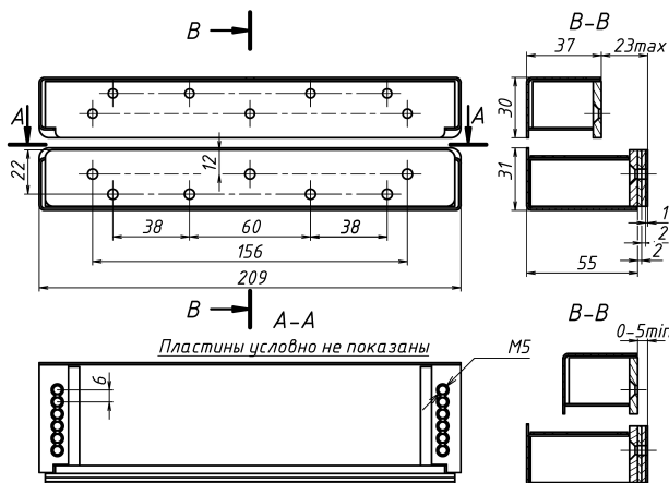
Рисунок 2 – Габаритно-установочные размеры комплекта МК 700S-PS
