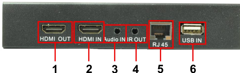
Рис. 3 Передатчик TLN-HiKM2, разъемы и индикаторы на задней панели
