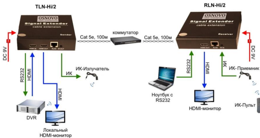
Рис.5 Схема подключения комплекта TLN-Hi/2+RLN-Hi/2 в режиме «точка-точка» через FE коммутатор
