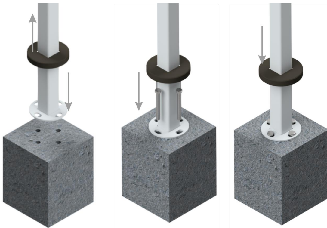
Рисунок 2-14 Монтаж стрелоуловителя
