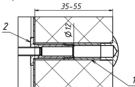
Рисунок 1 – Комплект поставки
