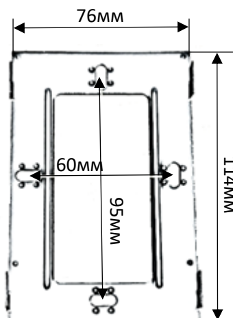
Монтажная пластина
