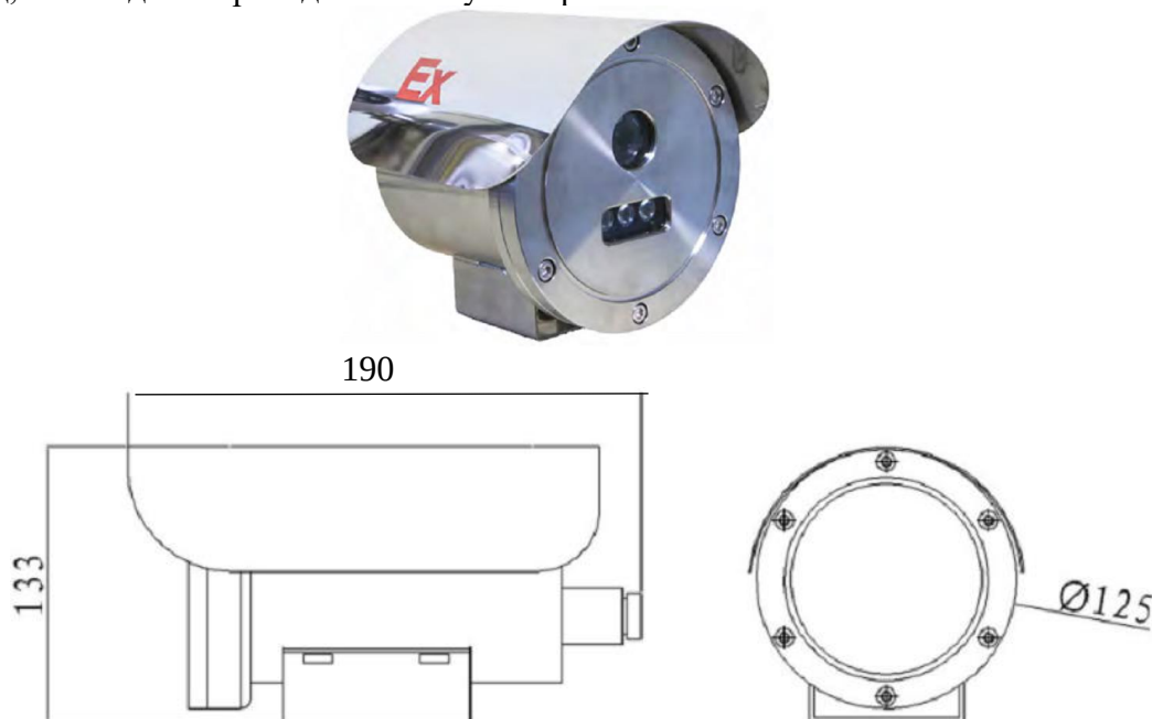
Рис. 1 – Общий вид видеокамеры с ИК-подсветкой модель Кондор-БК-Ex-100-Н/М
