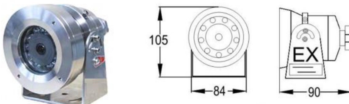
Рис. 1 – Общий вид мини видеокамеры с ИК-подсветкой модель Кондор-ВК-П-50-Н/М исп.1
