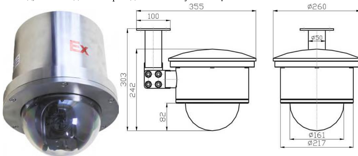
Рис. 1 – Общий вид видеокамеры модель Кондор-ВКК-Ex(исп.2)-Н/М
