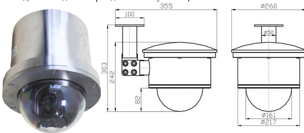
Рис. 1 – Общий вид видеокамеры модель Кондор-ВКК-П(исп.2) -Н/М
