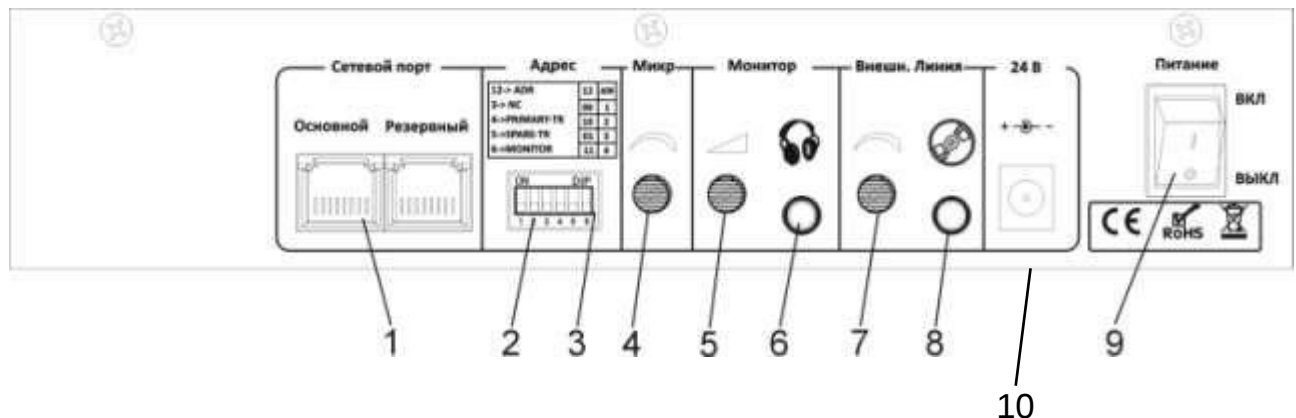
Рис. 3.3. Задняя панель микрофонной консоли LPA-EVA-RM
