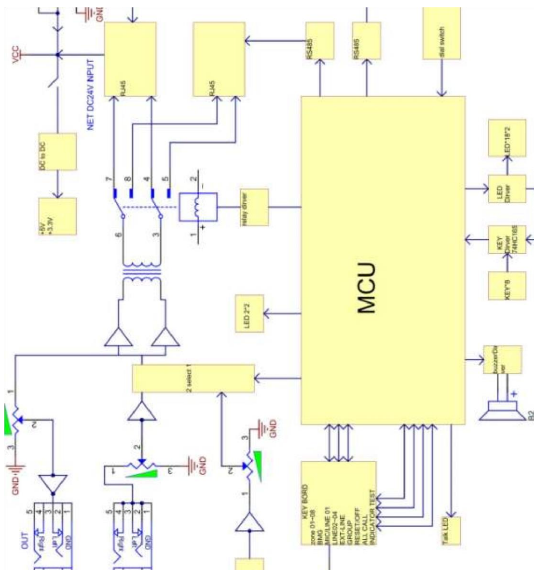
Рис. 5.1. Блок-схема микрофонной консоли LPA-EVA-RM
