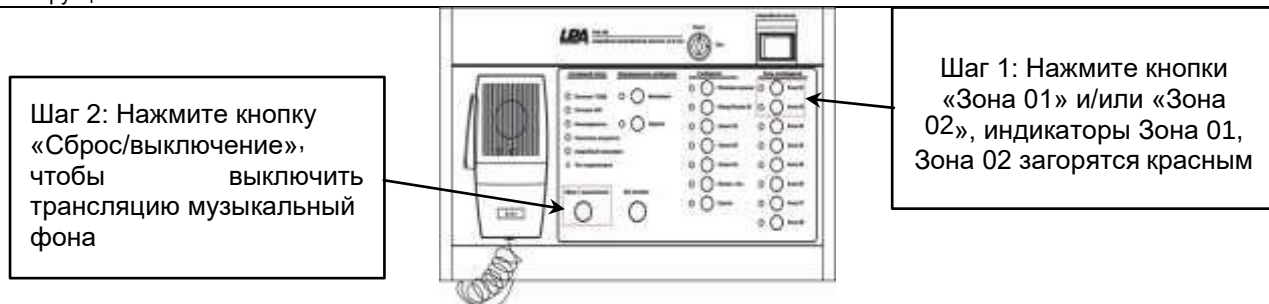
Рис. 4.7. Выключение трансляции фоновой музыки на микрофонной консоли LPA-EVA-FM
