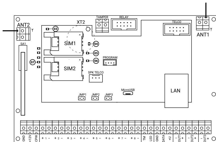
Рисунок 1. Лицевая сторона панели
