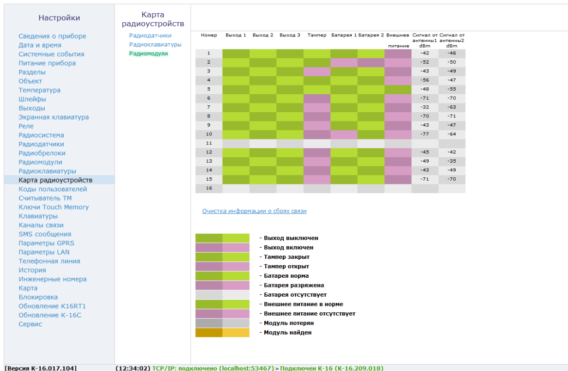
Рисунок 46. Карта радиоустройств: радиомодули
