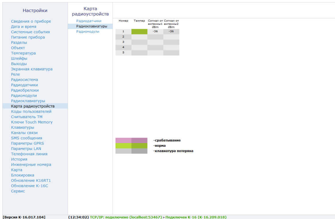
Рисунок 45. Карта радиоустройств: радиоклавиатуры
