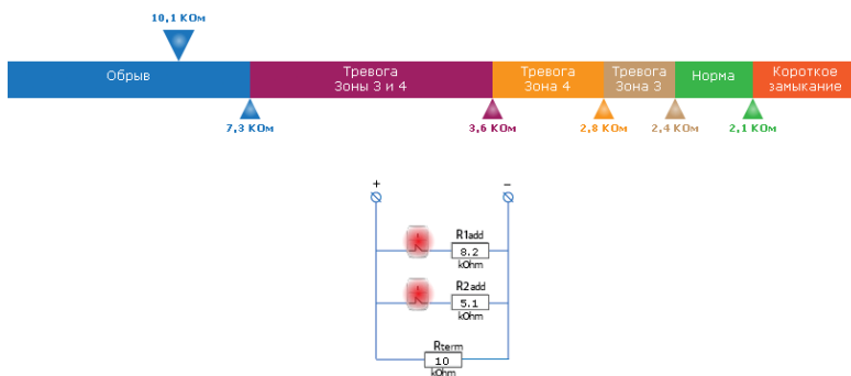
Рисунок 25. Шкала сопротивления резистивного шлейфа
