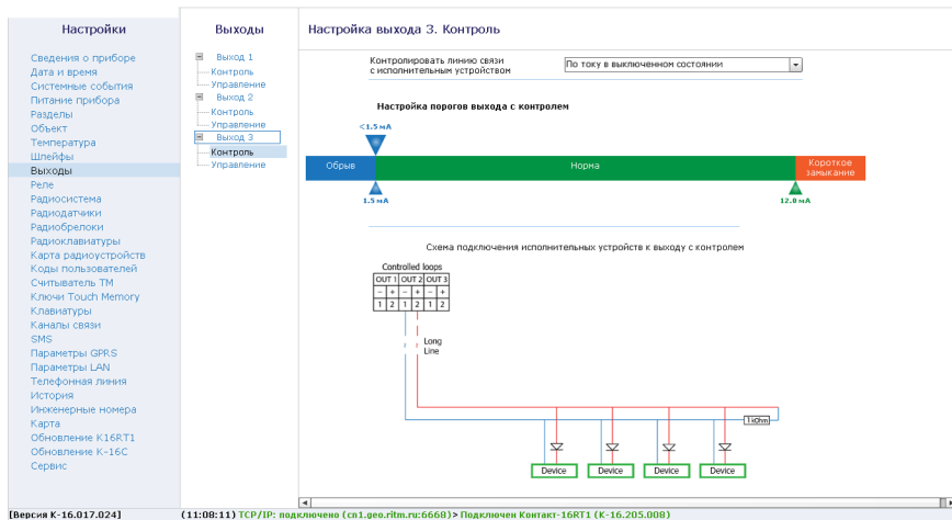
Рисунок 29. Контроль в выключенном состоянии
