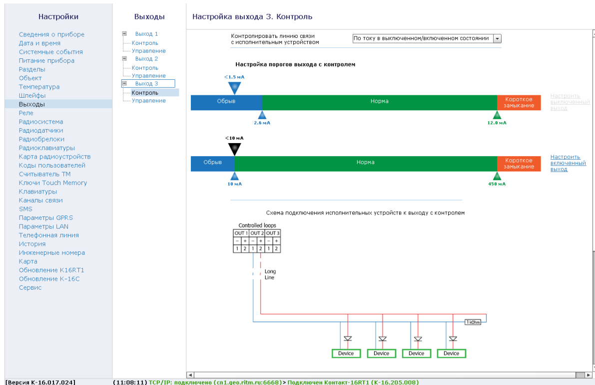
Рисунок 31. Контроль во включенном состоянии
