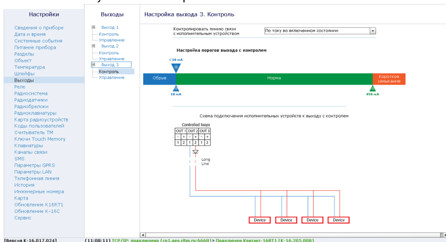
Рисунок 30. Контроль во включенном состоянии
