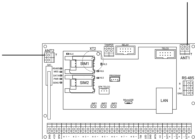
Рисунок 5. Схема подключения радиоканальных антенн
