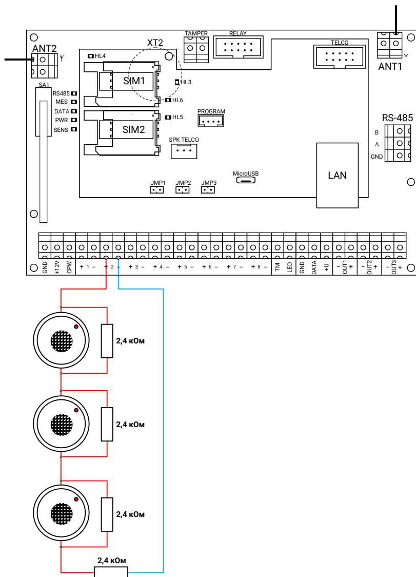
Рисунок 12. Схема подключения пожарных шлейфов
