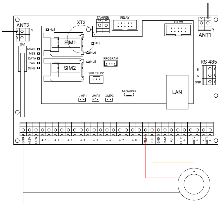
Рисунок 17. Схема подключения считывателя TM
