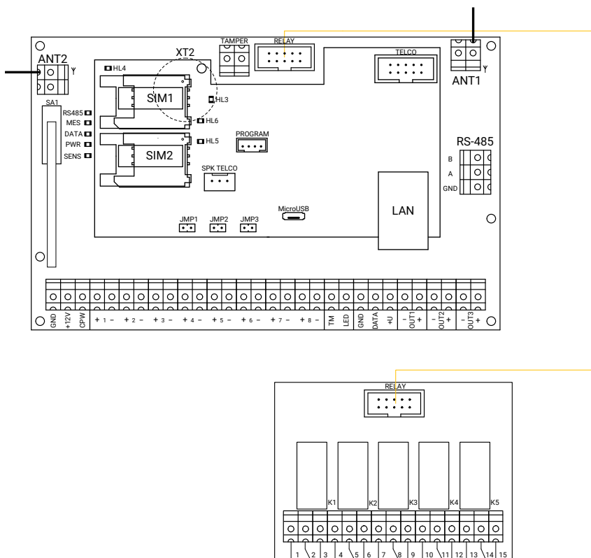
Рисунок 29. Схема подключения реле
