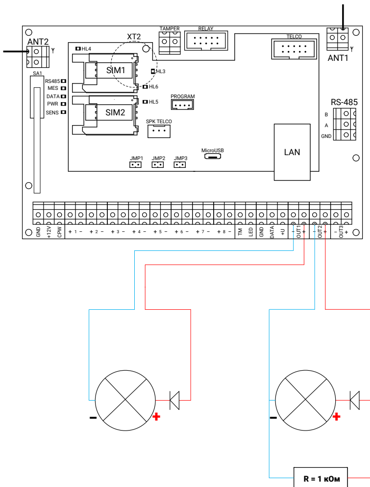
Рисунок 28. Схема подключения исполнительных устройств без использования плат контроля SCK16-1
