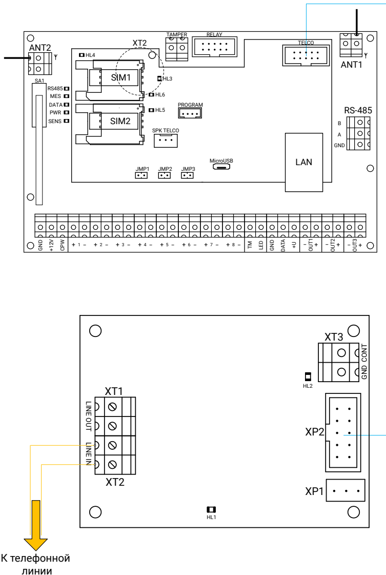
Рисунок 31. Схема подключения проводного модема K16
