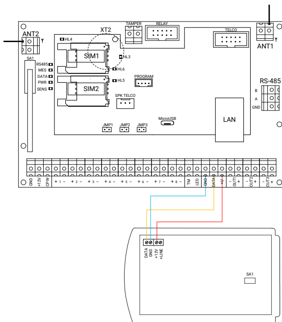
Рисунок 21. Схема подключения проводной клавиатуры
