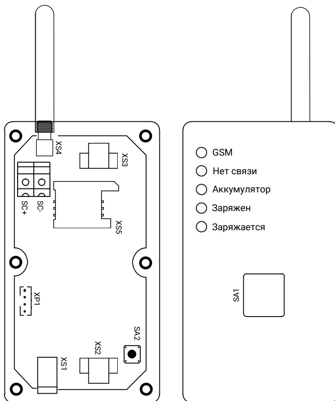
Рисунок 1. Внешний вид прибора
