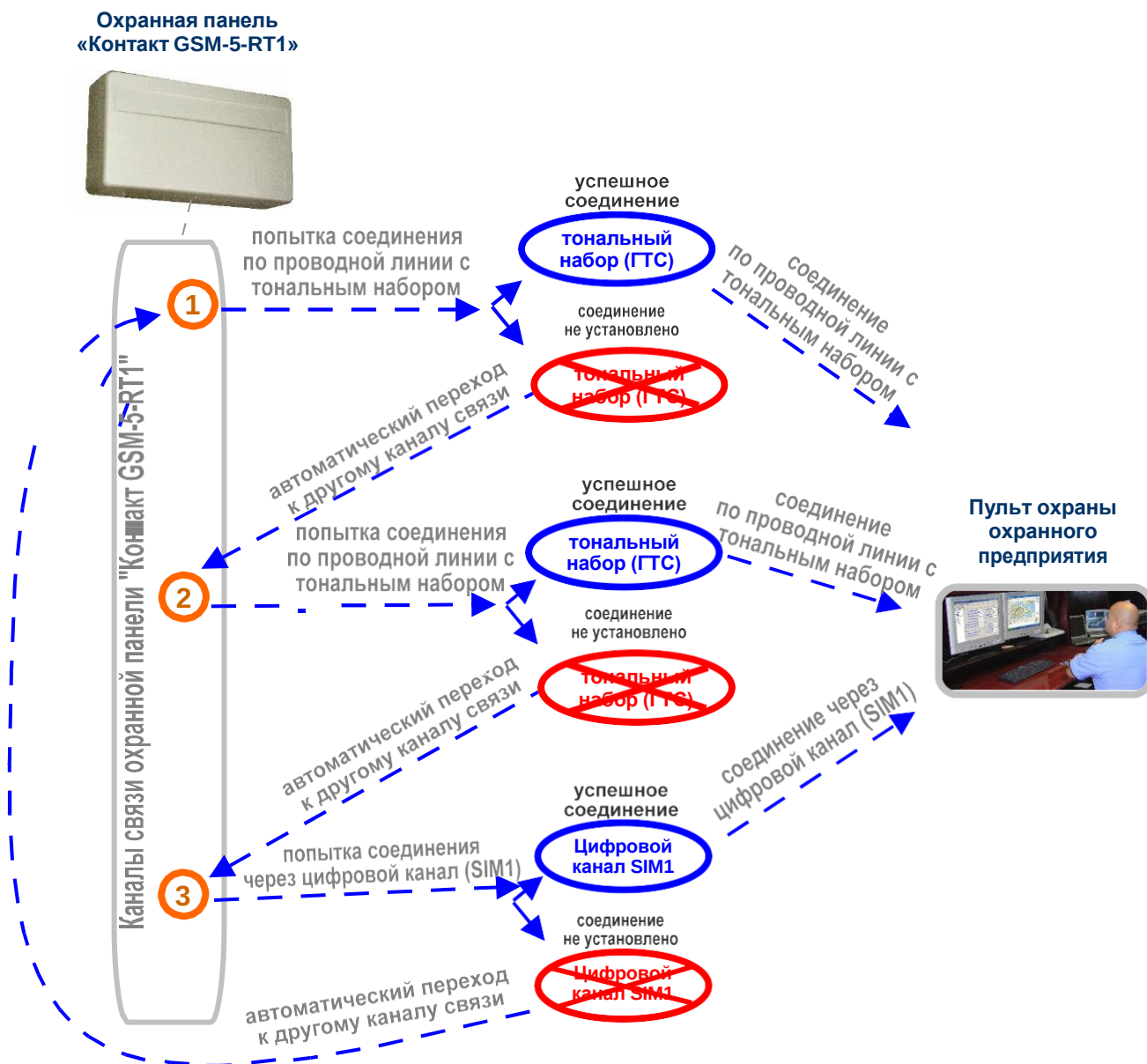
Рис.7.4. Приоритет каналов связи при работе «Контакт GSM-5-RT1» с одним охранным предприятием (в одном направлении связи).
