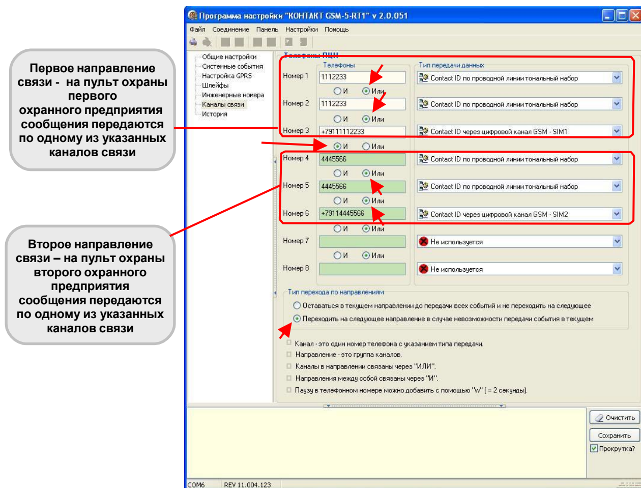
Рис.7.6. Настройка каналов связи для работы в режиме передачи сообщений «по событию» в двух направлениях связи. Программа Contact5RT1.exe, страница «Каналы связи».
