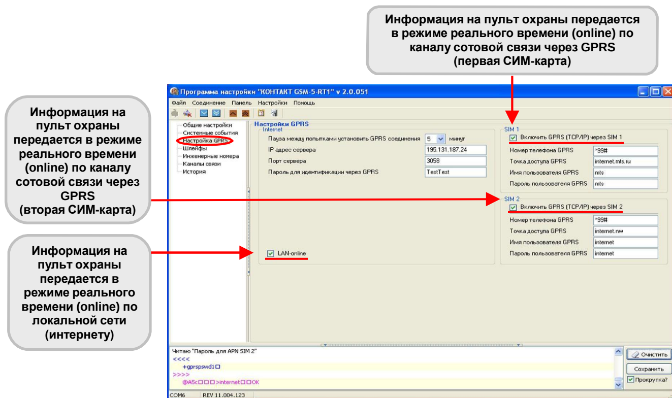
Рис.8.2. Настройка каналов связи для работы в режиме постоянного соединения в программе Contact5RT1.exe на странице «Настройки GPRS».
