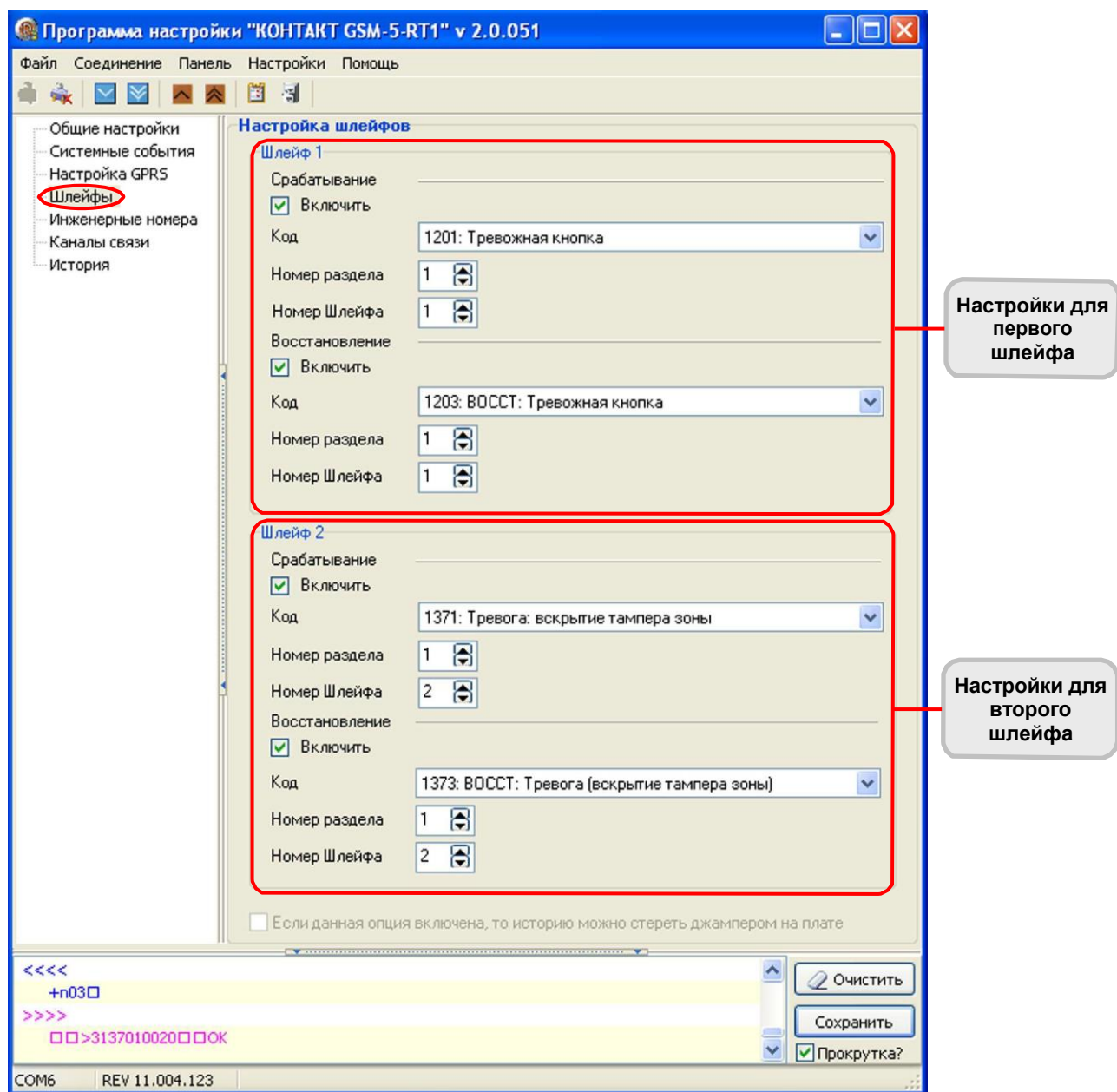
Рис.5.13. Страница «Шлейфы».
