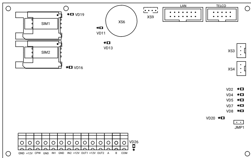
Рисунок 1. Плата панели
