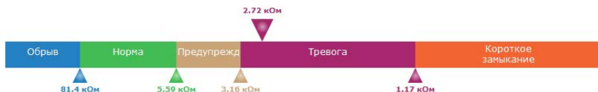
Рисунок 23. Шкала порогов пожарного шлейфа
