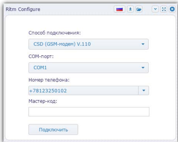
Рисунок 9. Настройка CSD-соединения в программе Ritm Configure
