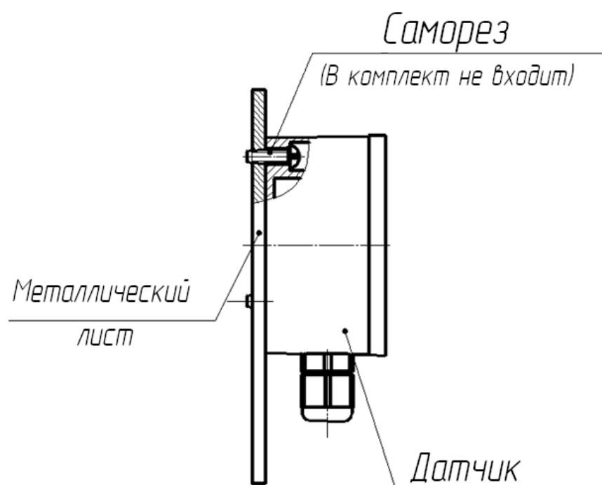
Рисунок 2.1 – в) Крепление датчика к металлическому листу
