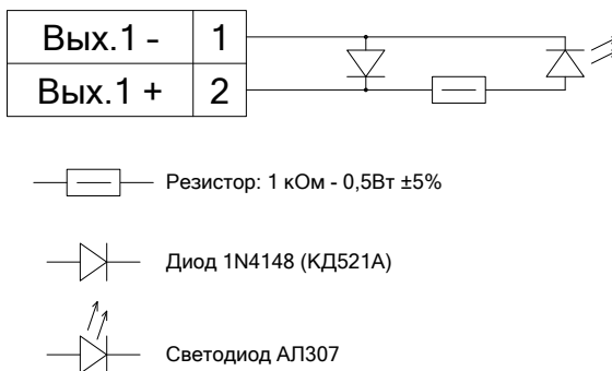
Рисунок 6. Схема имитатора пусковой цепи.
