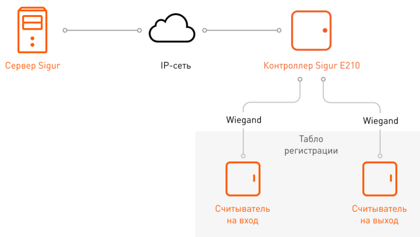
Вариант подключения в конфигурации «Терминал учёта рабочего времени».
