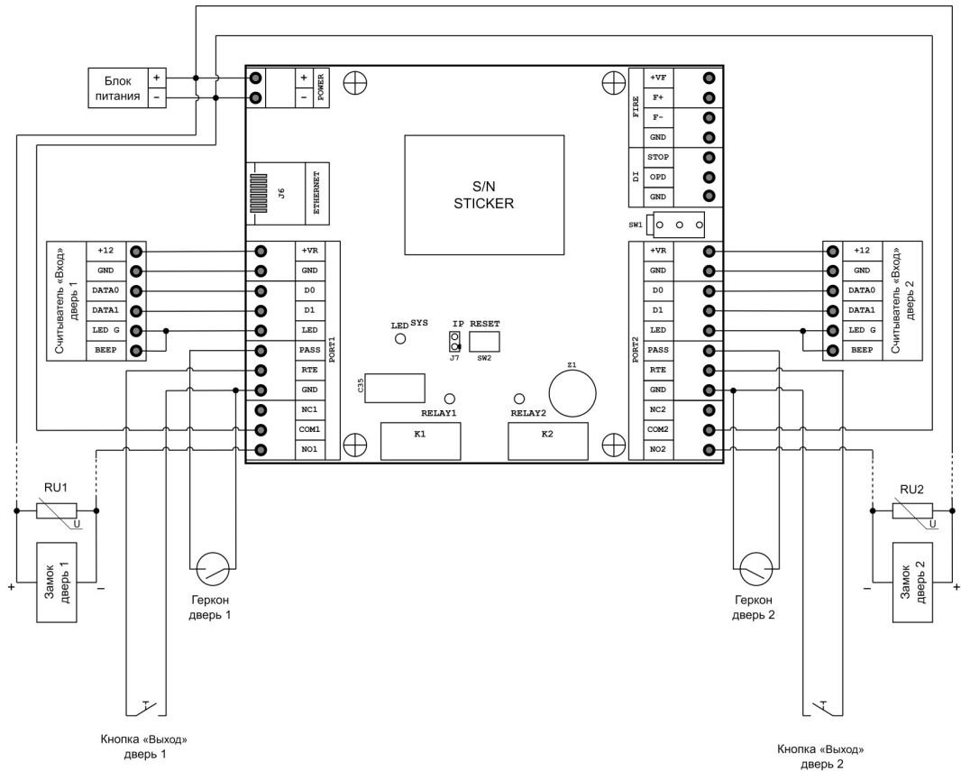
Пример подключения двух дверей.
