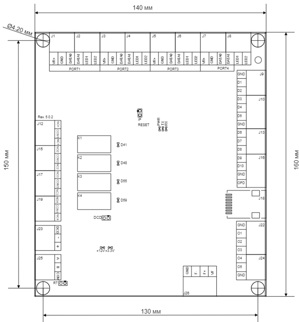
Схема расположения основных элементов на плате контроллера E510 и E510 UPS.
