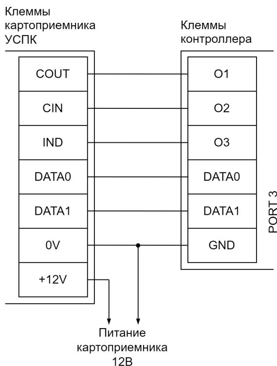
Пример подключения УСПК в направлении «Выход».
