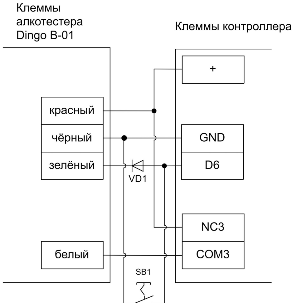
Подключение Динго В-01 к турникету.
