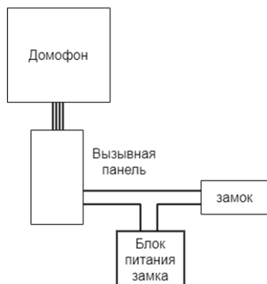
Исходная схема подключения
