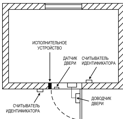
Рисунок 3 – Пункт прохода с контролем входа/выхода
