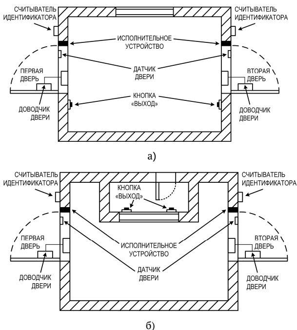
Рисунок 4 – Пункт прохода: шлюз
