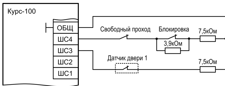
Рисунок 13 – Схема подключения ШС для конфигурации «2ШС+1ТД (Пункт прохода)» с управлением нормально замкнутыми контактами
