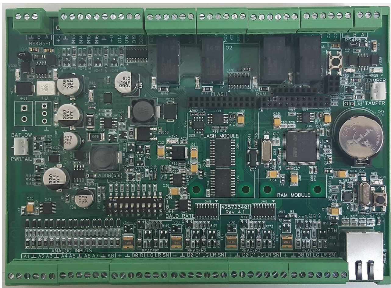
Рисунок 5. Контроллер ЛКД-КС-150000-02 в сборе
