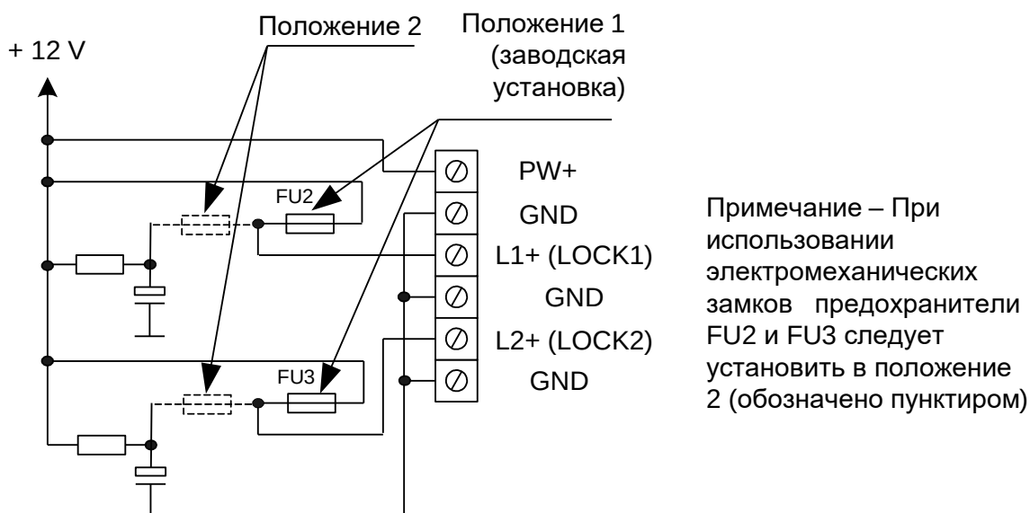
Рисунок 4. Подключение накопительной RC-цепочки для питания электромеханических замков на коммутационной плате источника.
