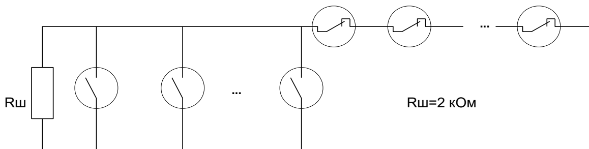
Рисунок 15. Подключение устройств с нормально замкнутыми и нормально разомкнутыми контактами к аналоговым входам, с использованием оконечного резистора
