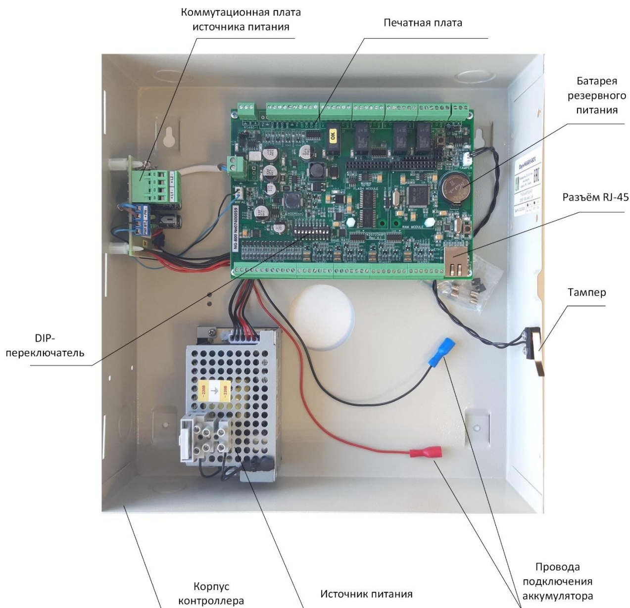
Рисунок 6. Контроллер ЛКД-КС-150000-01 в сборе
