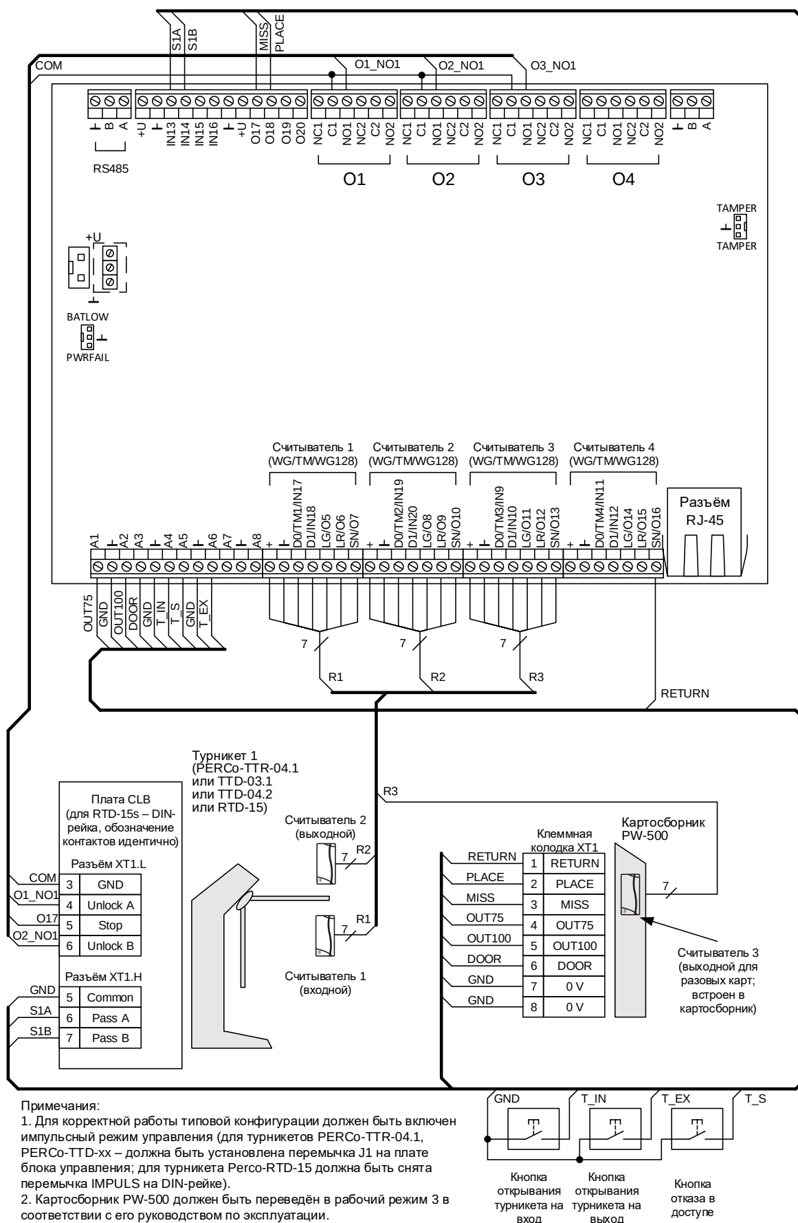
Рисунок 21. Схема подключения турникета PERCo совместно с картосборником PW500
