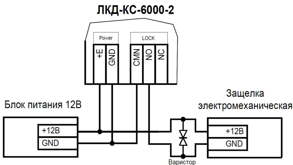
Рисунок 11. Схема подключения отпираемой напряжением защелки
