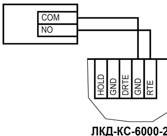
Рисунок 14. Схема подключения кнопки запроса на выход
