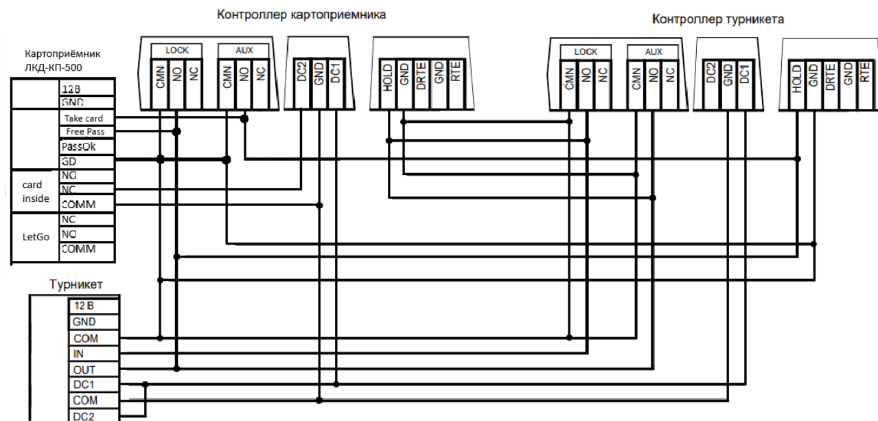
Рисунок 10. Схема подключения картоприемника ЛКД-КП-500 к контроллеру
