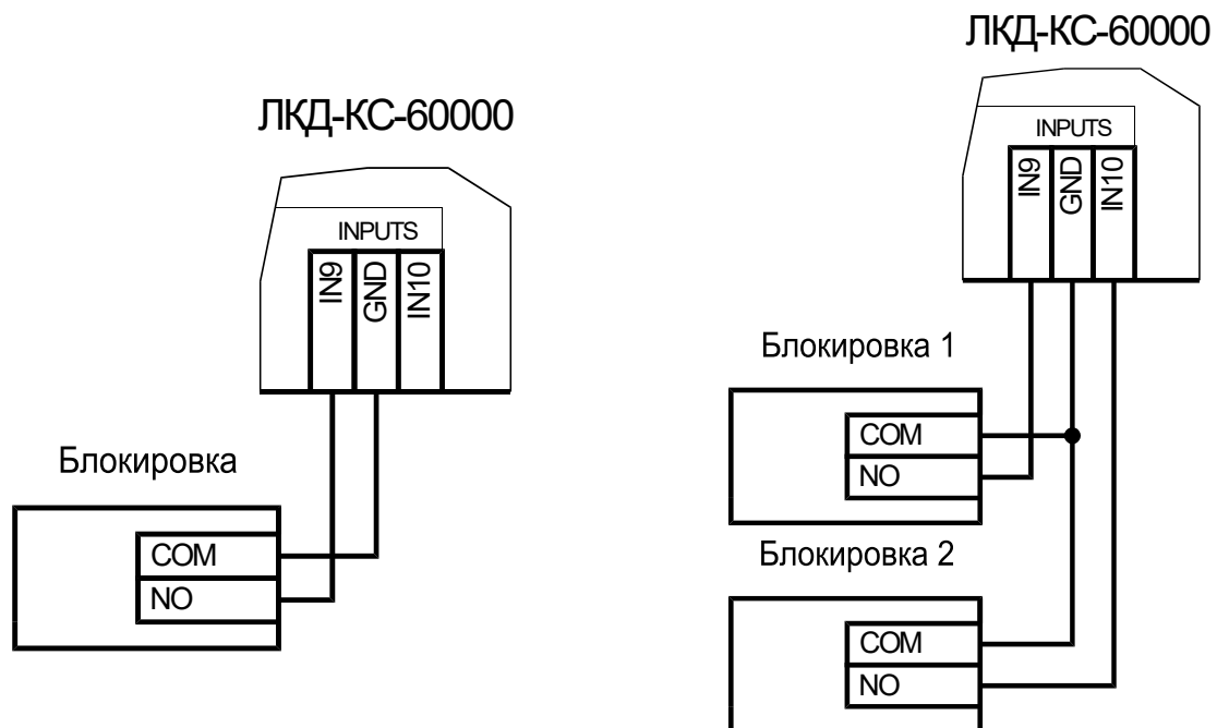
Рисунок 22. Схемы подключения блокировки контроллера
