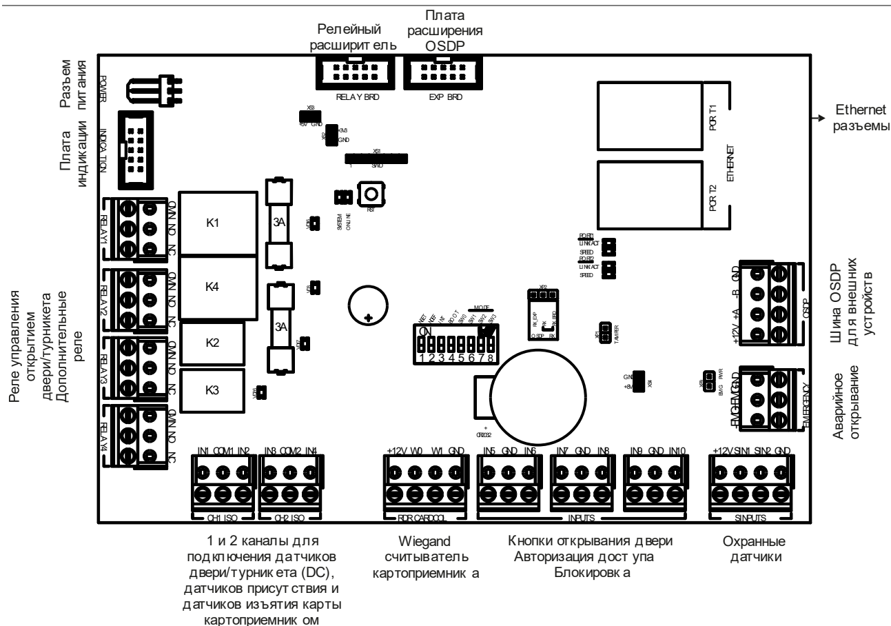
Рисунок 2. Схема платы контроллера ЛКД-КС-60000
