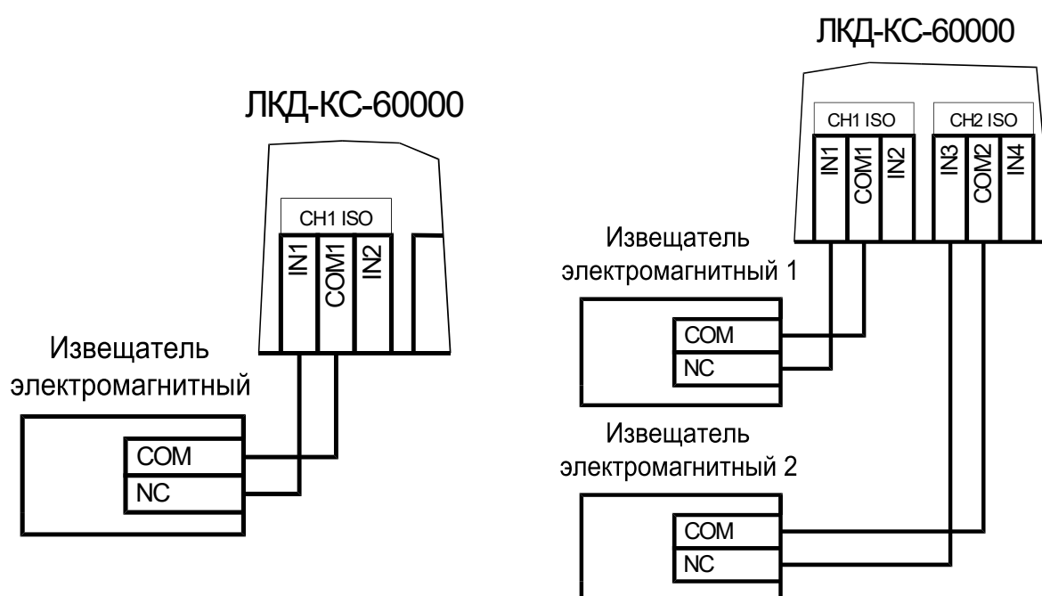
Рисунок 16. Схемы подключения дверного контакта для точки прохода типа «дверь»
