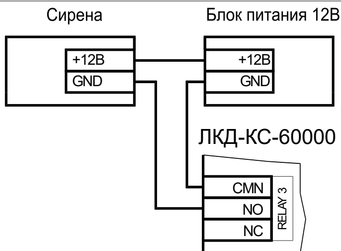
Рисунок 24. Схема подключения сирены к RELAY 3
