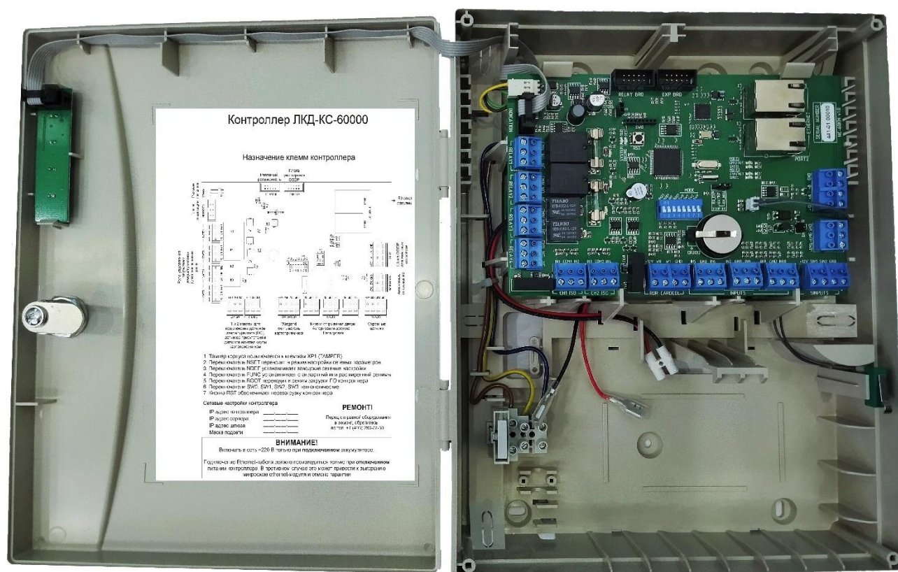
Рисунок 1. Контроллер ЛКД-КС-60000 в корпусе
