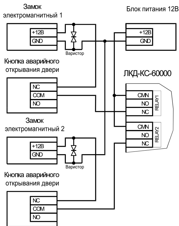
Рисунок 11. Схема подключения двух замков, запираемых напряжением
