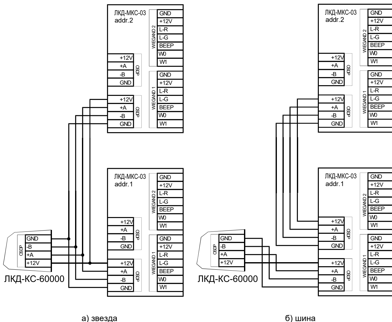
Рисунок 10. Подключение преобразователей Wiegand-OSDP
