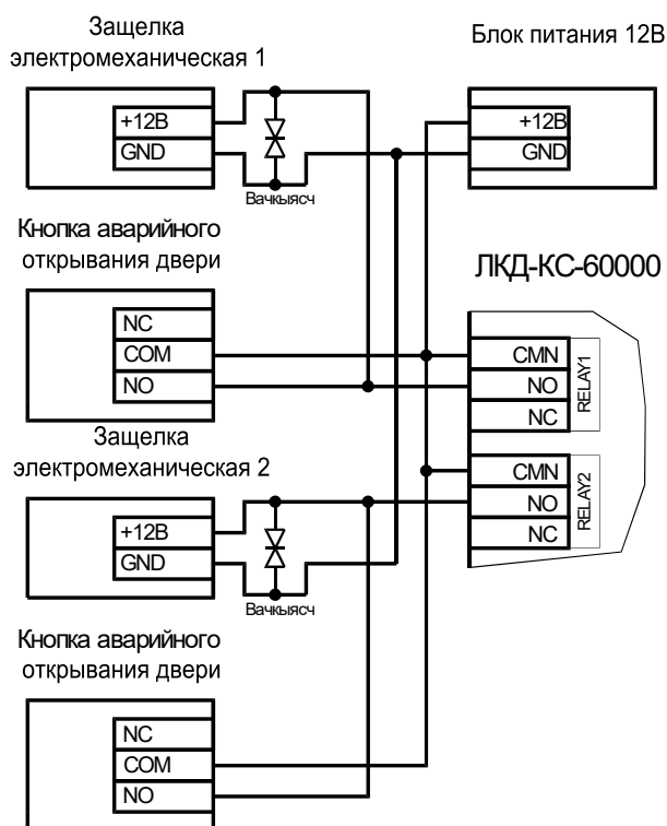
Рисунок 12. Схема подключения 2 защелок, отпираемых напряжением
