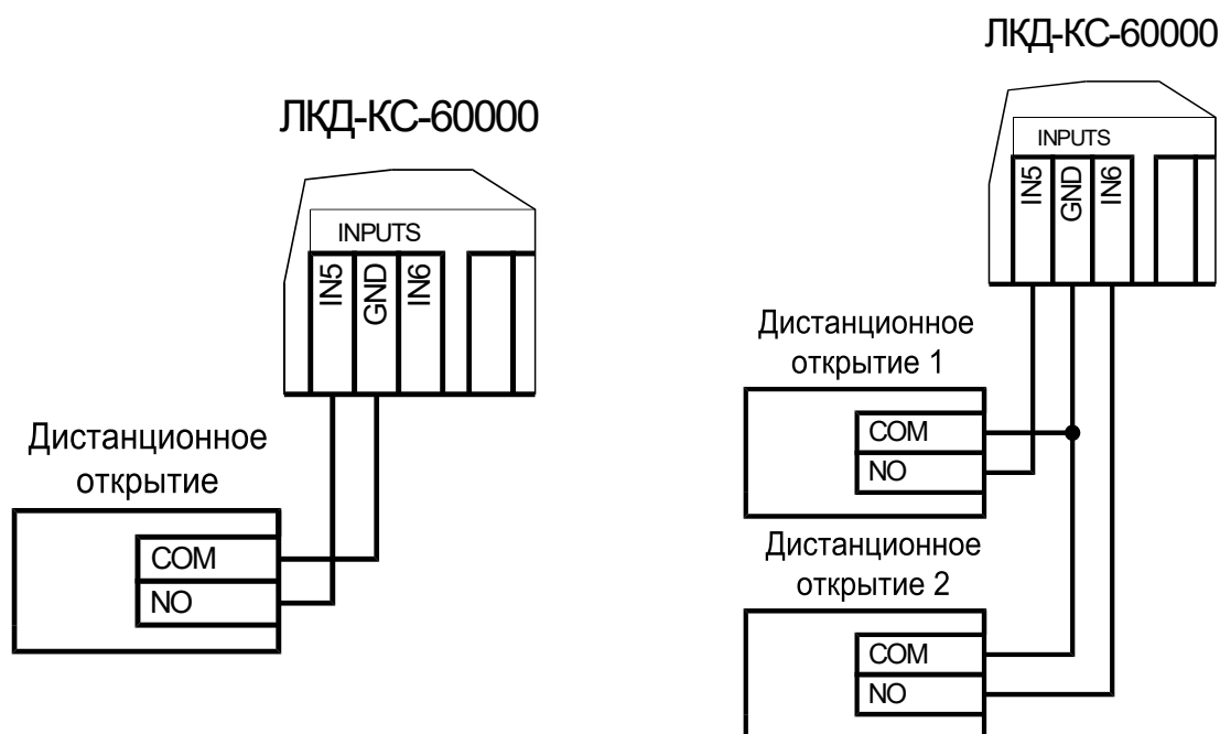
Рисунок 15. Схемы подключения кнопок удаленного открывания дверей
