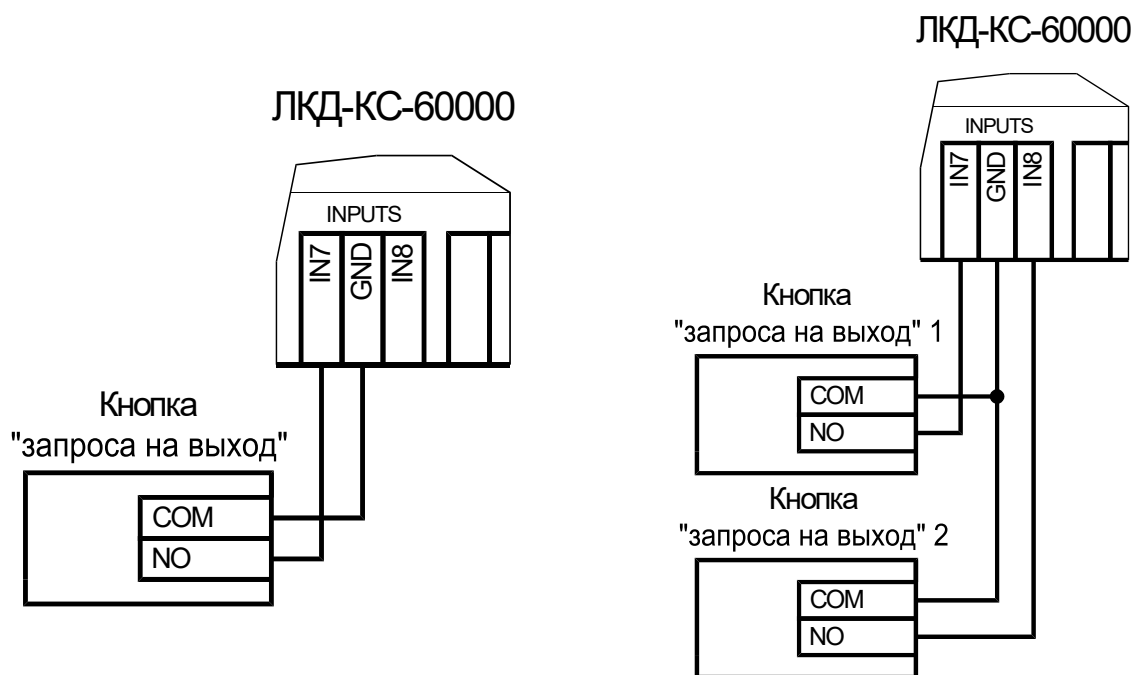
Рисунок 14. Схемы подключения кнопок запроса на выход
