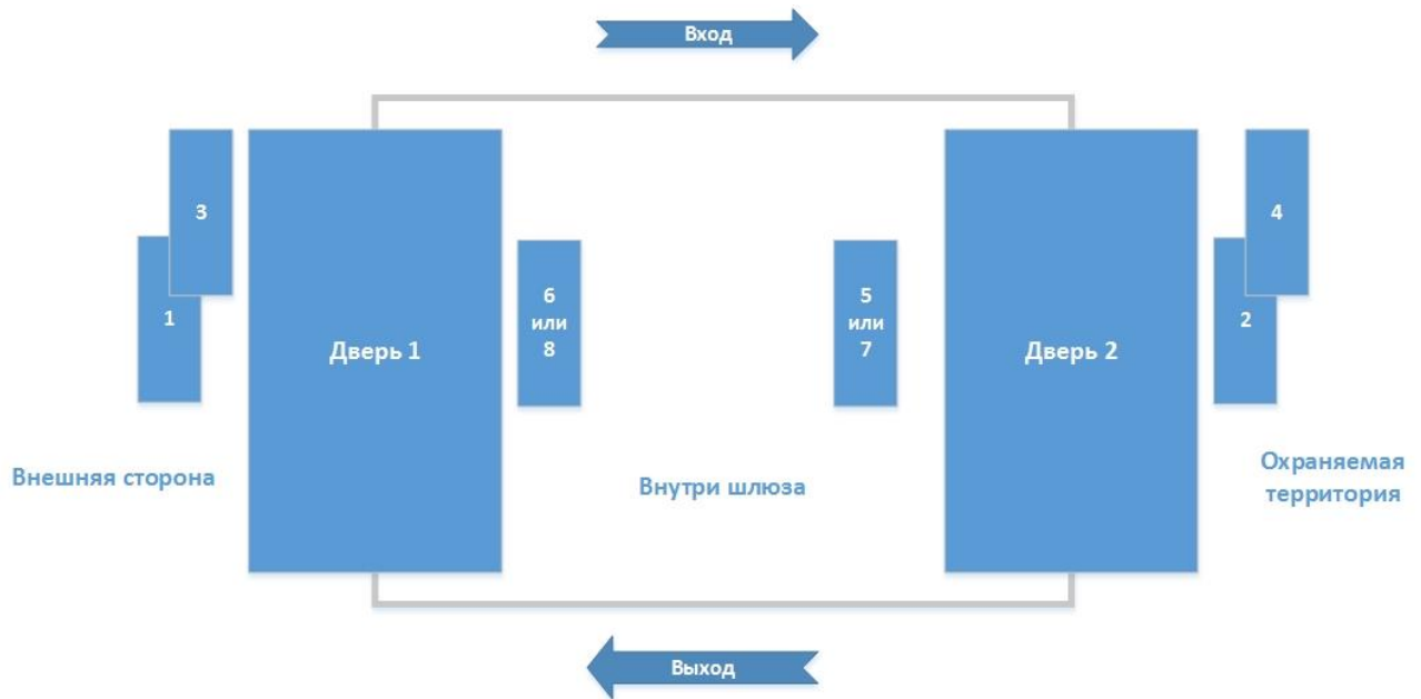
Рисунок 7. Адреса считывателей шлюза
