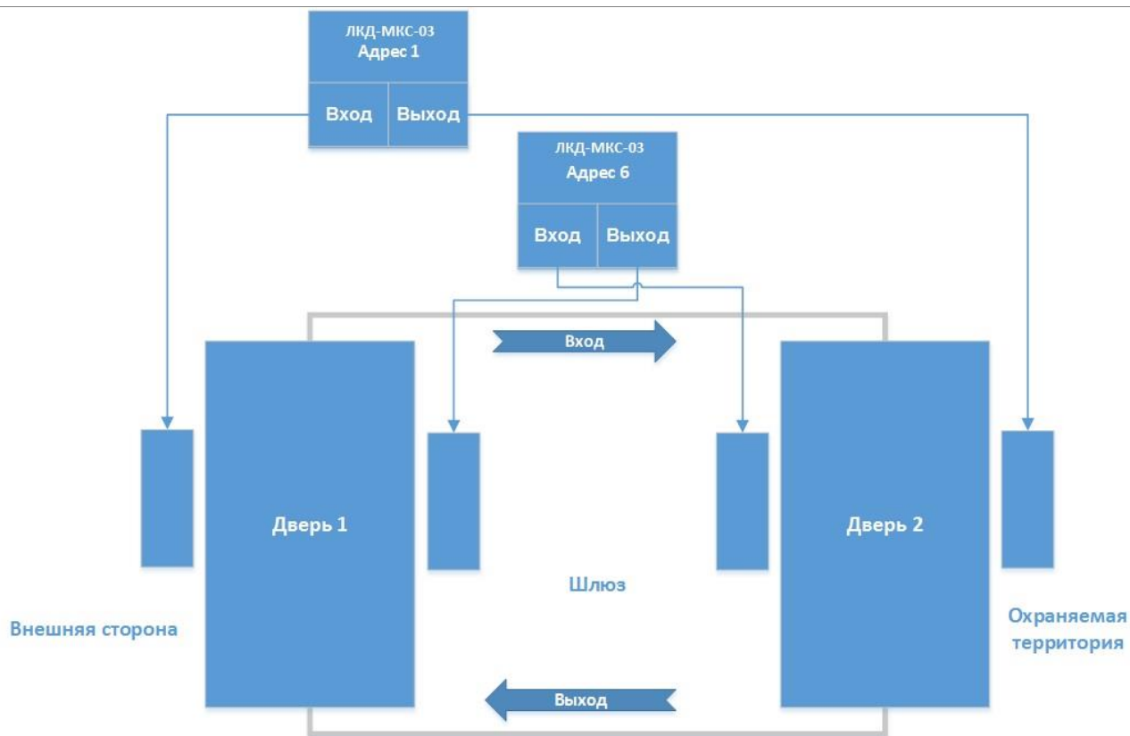
Рисунок 8. Адреса считывателей шлюза, подключенных посредством преобразователей ЛКД-МКС-03
