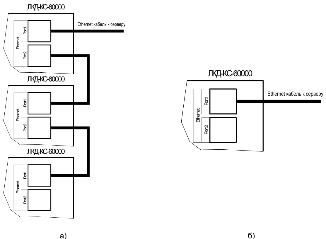
Рисунок 30. Подключение контроллеров к сети Ethernet:
