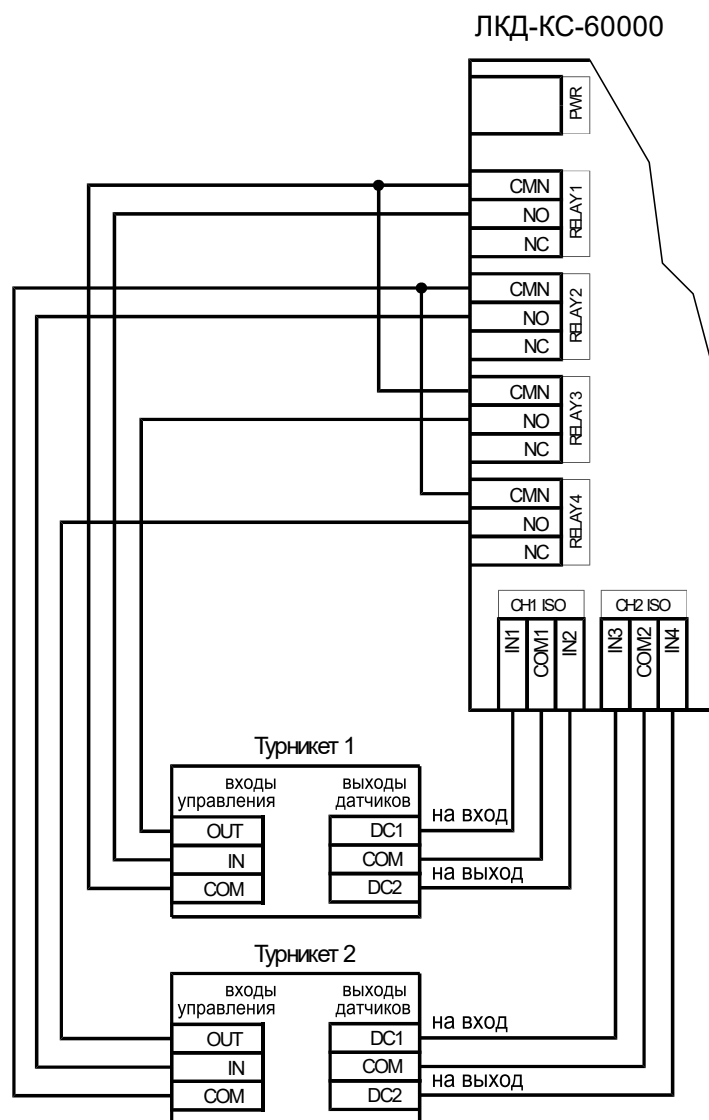
Рисунок 18. Схема подключения 2 турникетов
