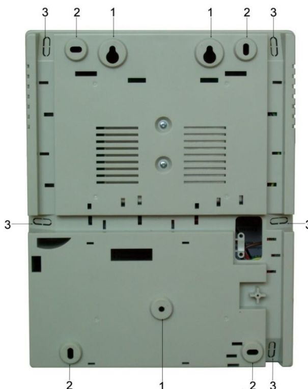
Рисунок 3. Монтажные отверстия
