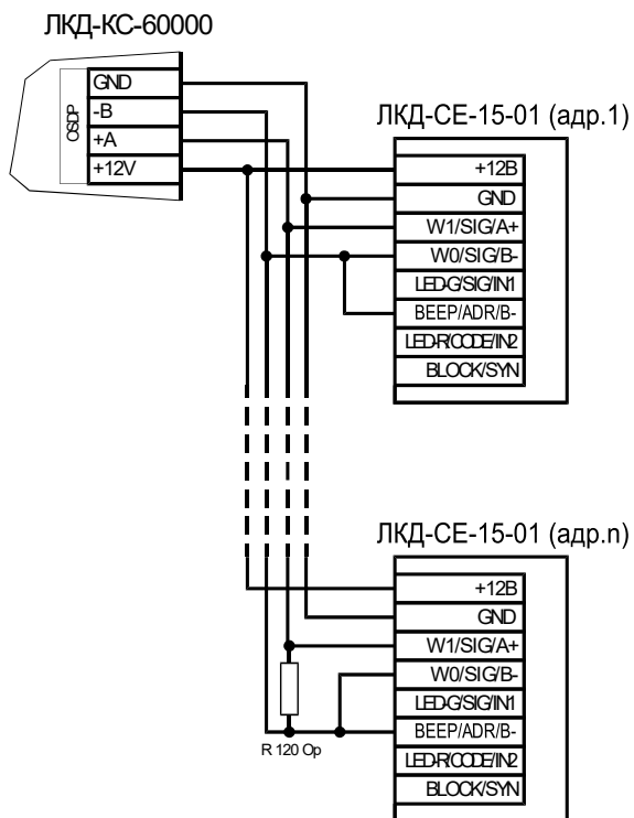
Рисунок 9. Подключение OSDP считывателей
