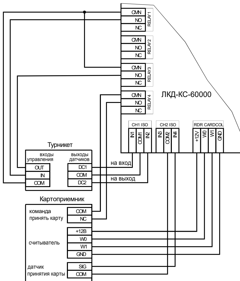
Рисунок 17. Схема подключения турникета и картоприемника
