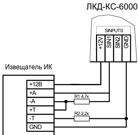
Рисунок 20. Схема подключения охранного датчика с контролем состояния линии
