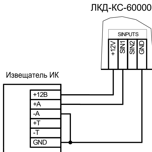
Рисунок 21. Схема подключения охранного датчика без контроля состояния линии
