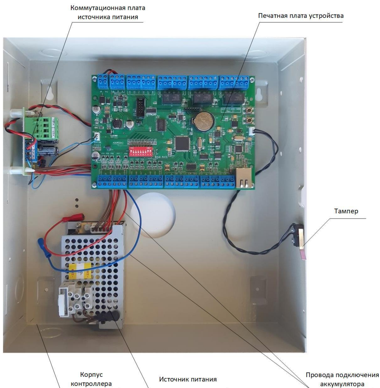
Рисунок 6. Контроллер ЛКД-КС-75000-01 в сборе
