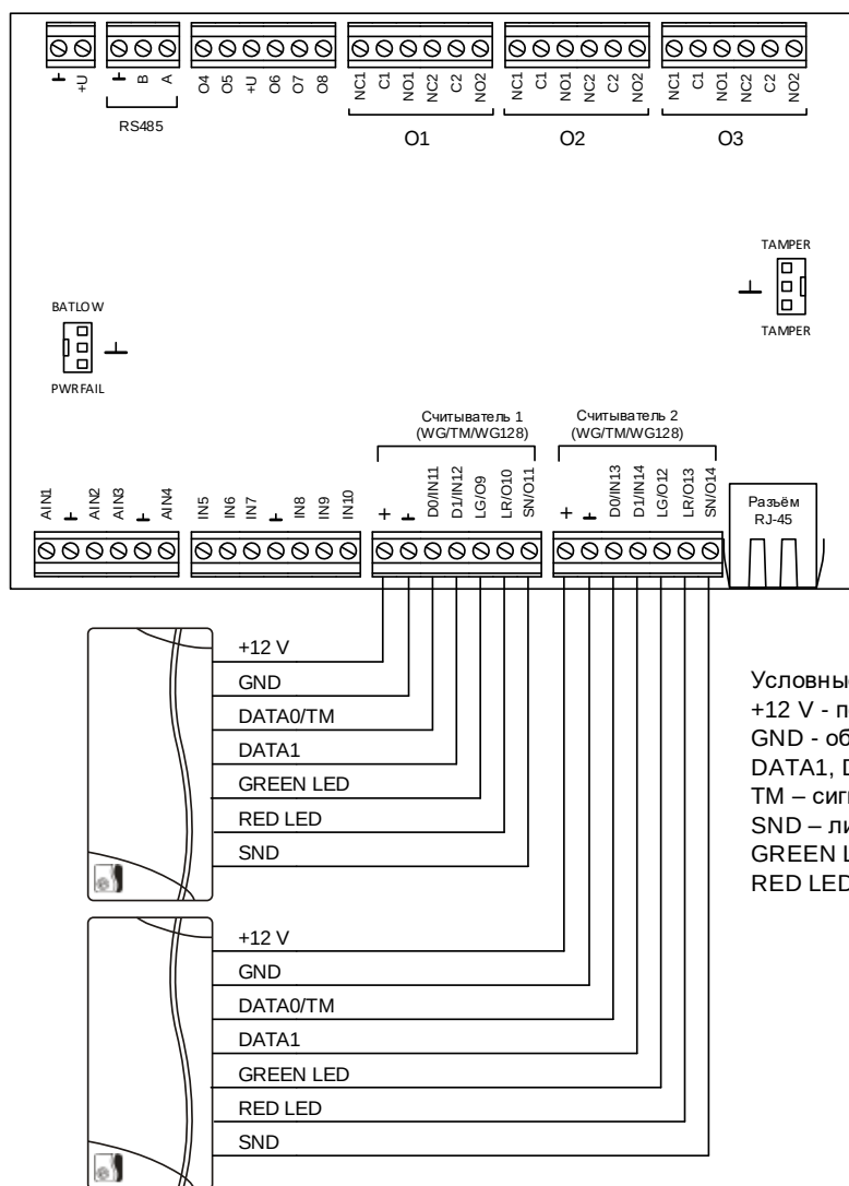
Рисунок 9. Схема подключения считывателей по интерфейсу Wiegand или Touch Memory
