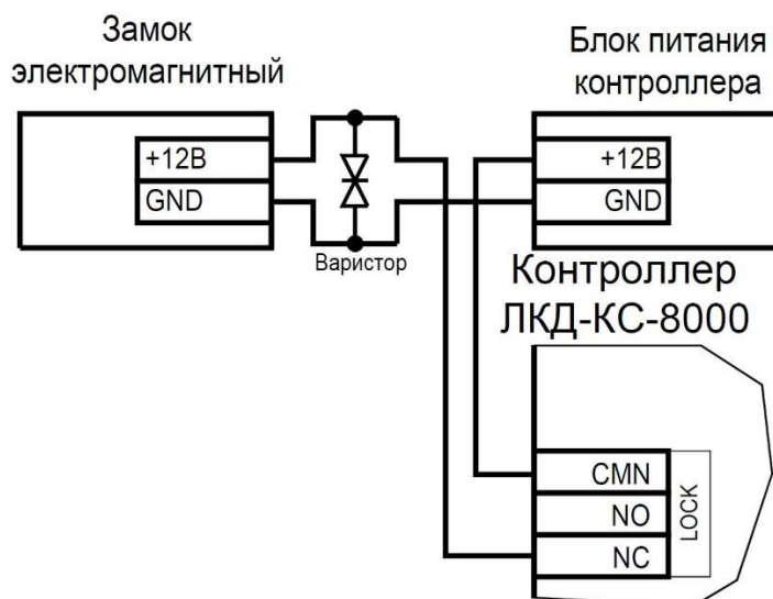
Рисунок 10. Схема подключения замка, запираемого напряжением
