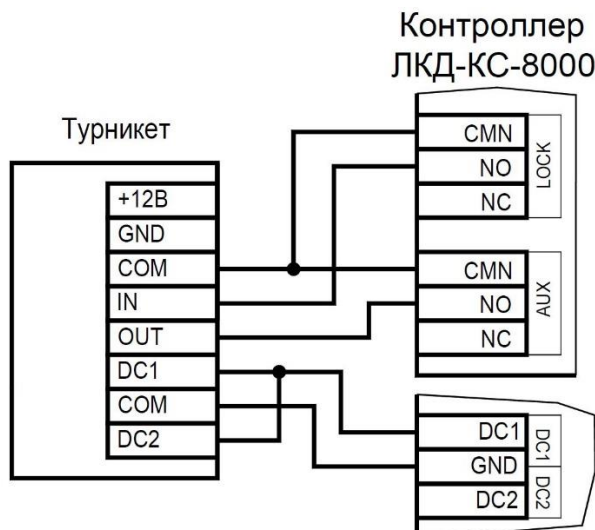
Рисунок 13. Схема подключения контроллера к турникету
