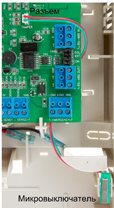
Рисунок 20. Подключение тампера корпуса
