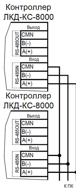
Рисунок 26. Пример соединения контроллеров по топологии «Звезда»
