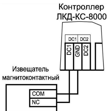
Рисунок 16. Схема подключения дверного контакта
