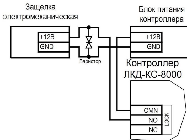
Рисунок 7. Схема подключения защелки, отпираемой напряжением
