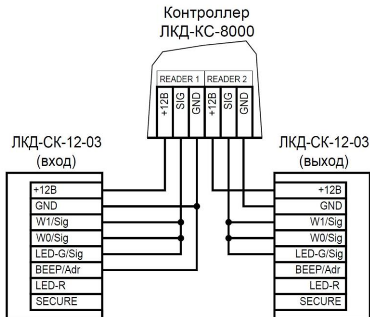
Рисунок 8. Схема подключения считывателей к контроллеру двумя кабелями
