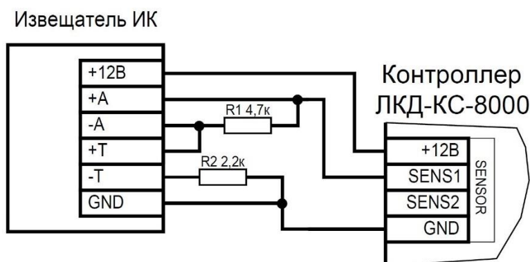
Рисунок 17. Схема подключения охранного датчика с контролем состояния линии
