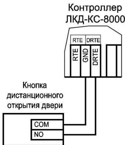
Рисунок 15. Схема подключения кнопки дистанционного открывания двери
