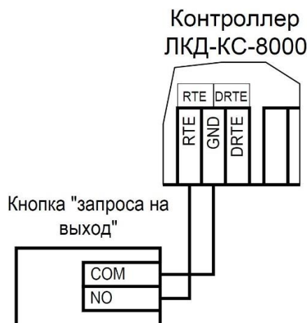
Рисунок 14. Схема подключения кнопки запроса на выход
