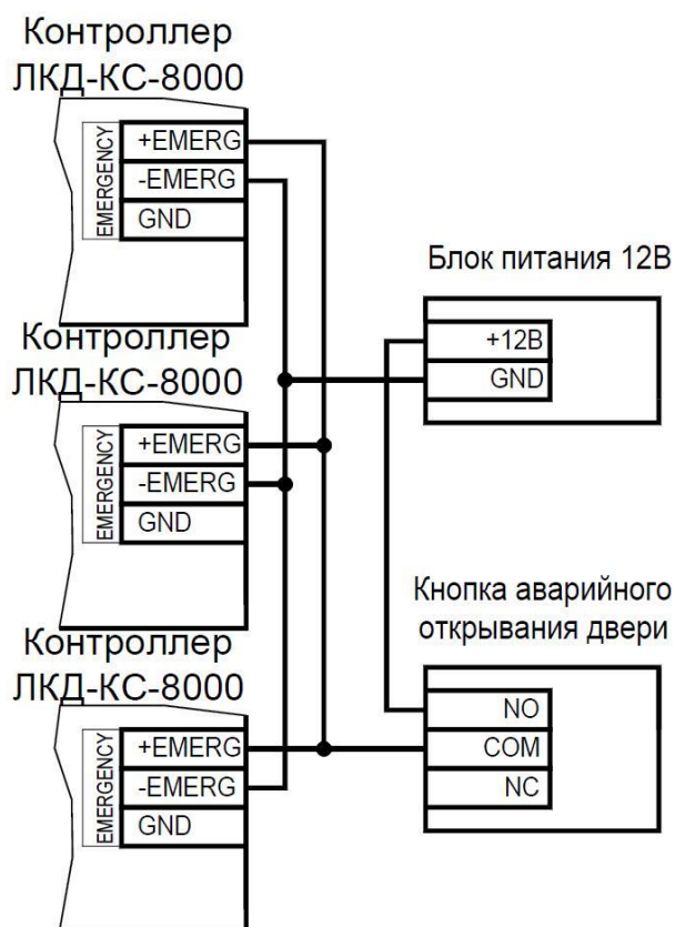
Рисунок 22. Схема подключения одной аварийной кнопки к нескольким контроллерам
