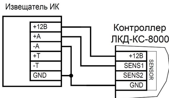
Рисунок 18. Схема подключения охранного датчика без контроля состояния линии
