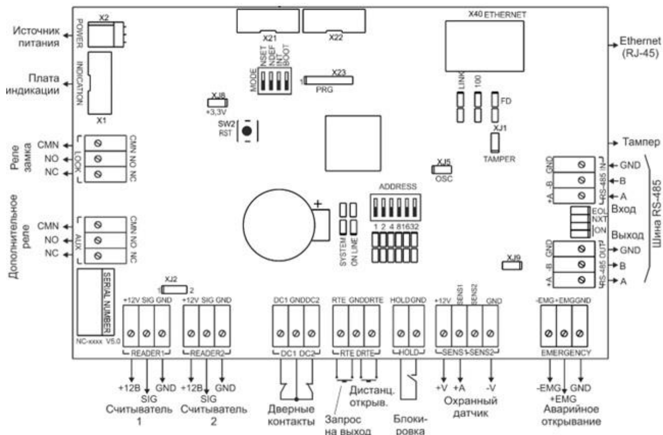
Рисунок 2. Схема платы контроллера ЛКД-КС-8000.
