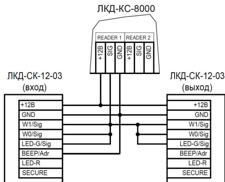
Рисунок 7. Схема подключения считывателей к контроллеру одним кабелем
