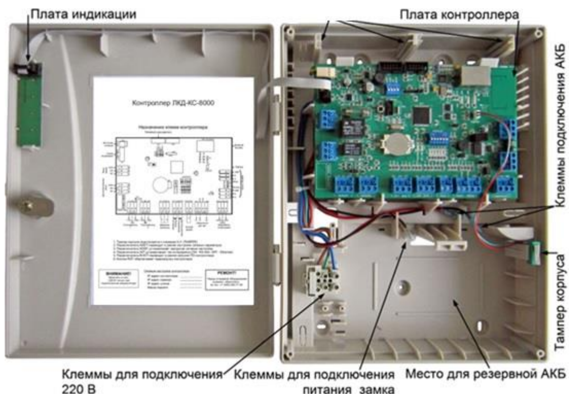
Рисунок 1. Открытый корпус с платой контроллера
