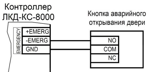
Рисунок 21. Схема подключения кнопки аварийного выхода к одному контроллеру
