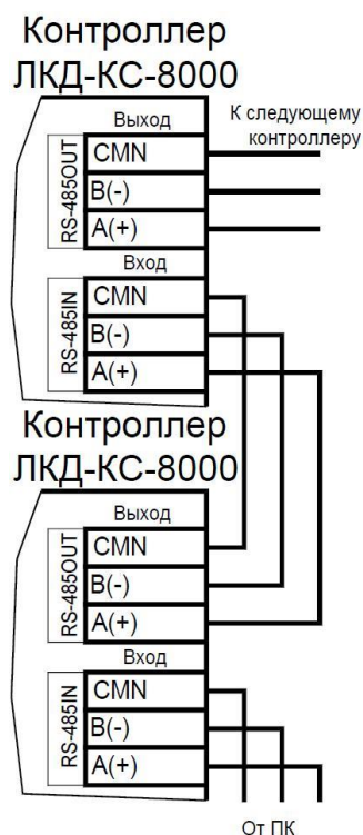
Рисунок 25. Схема соединения контроллеров по топологии «Шина»
