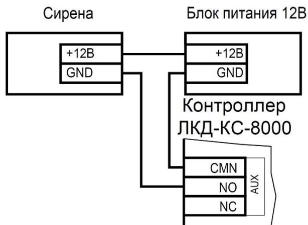
Рисунок 19. Схема подключения сирены к дополнительному реле
