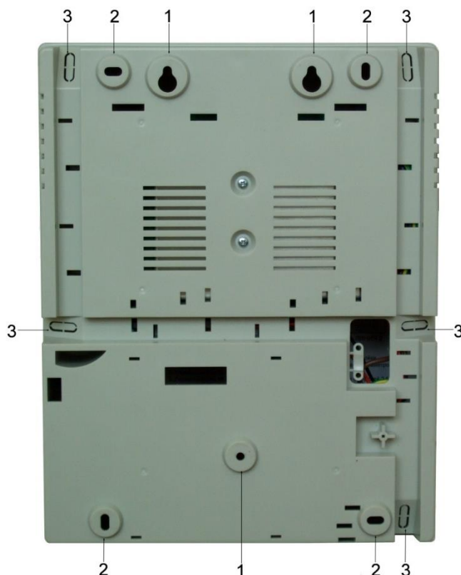
Рисунок 4. Монтажные отверстия
