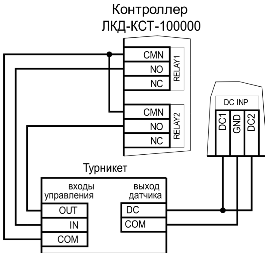
Рисунок 16. Схема подключения одного датчика проворота турникета
