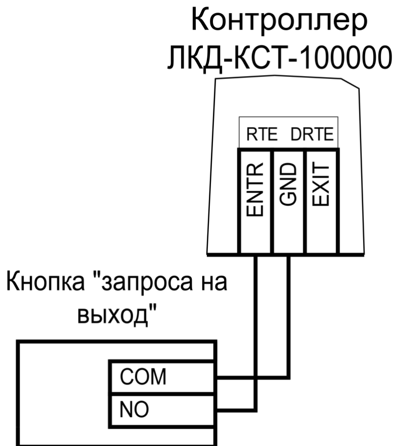
Рисунок 14. Схема подключения кнопки удаленного открывания двери
