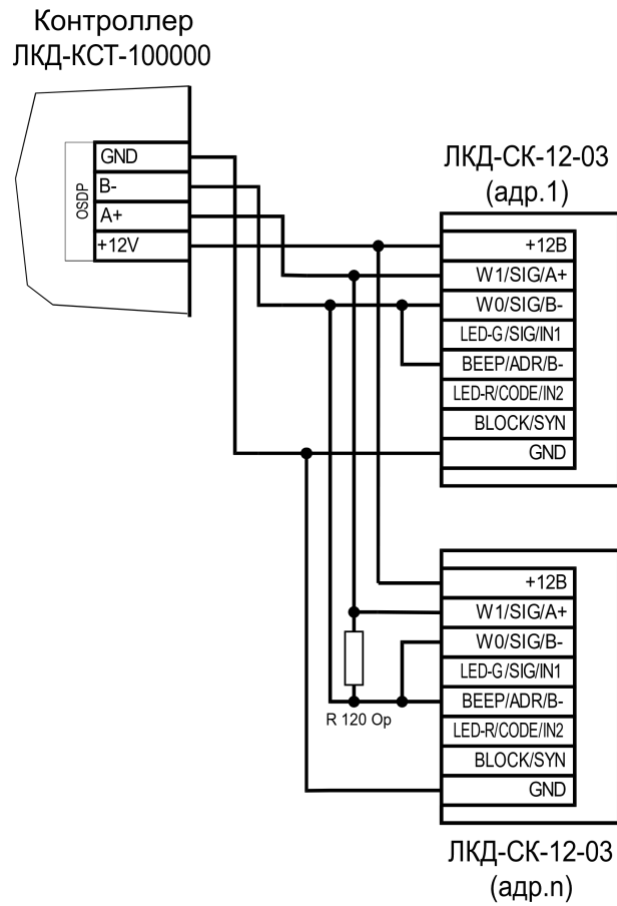
Рисунок 7. Подключение OSDP считывателей
