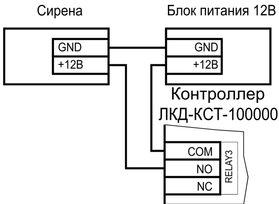
Рисунок 22. Схема подключения сирены к RELAY 3
