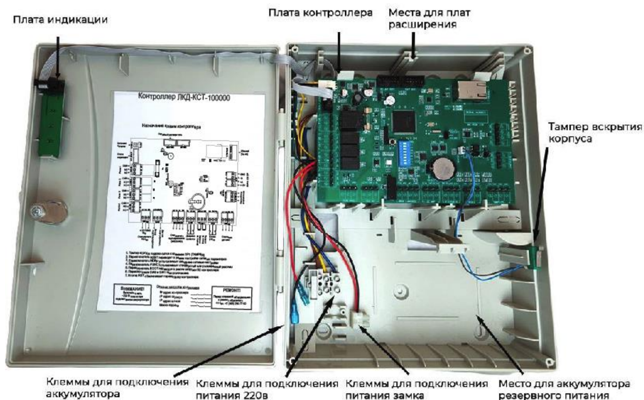
Рисунок 1. Открытый корпус с платой контроллера ЛКД-КСТ-100000
