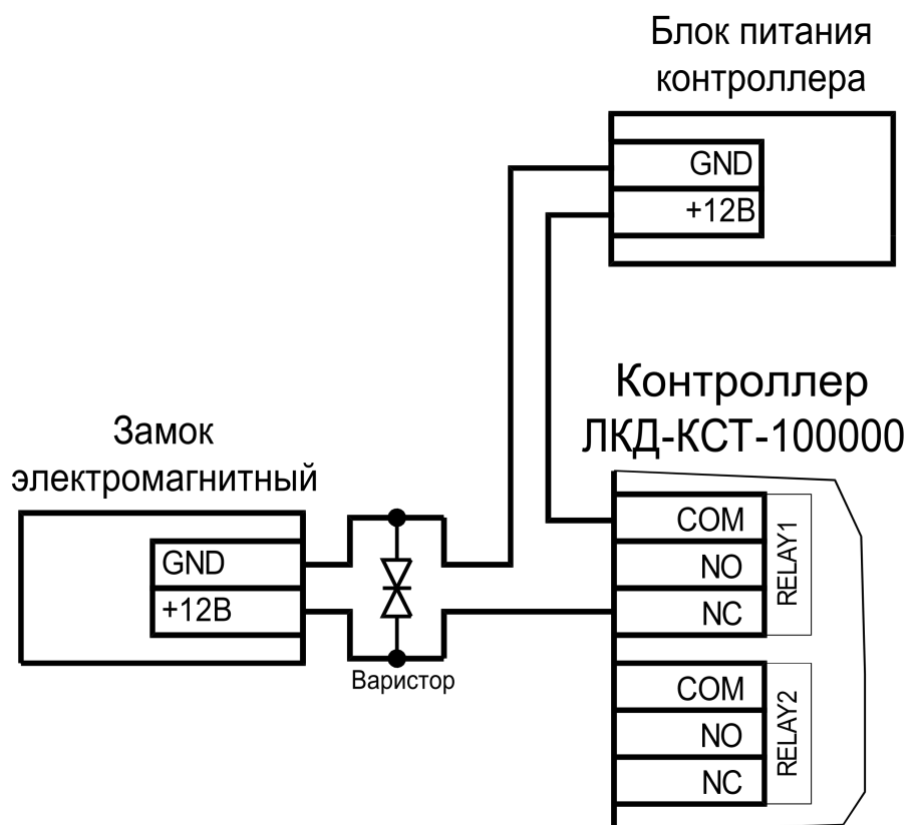
Рисунок 10. Схема подключения замка, запираемого напряжением
