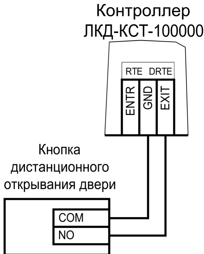
Рисунок 13. Схема подключения кнопки запроса на выход
