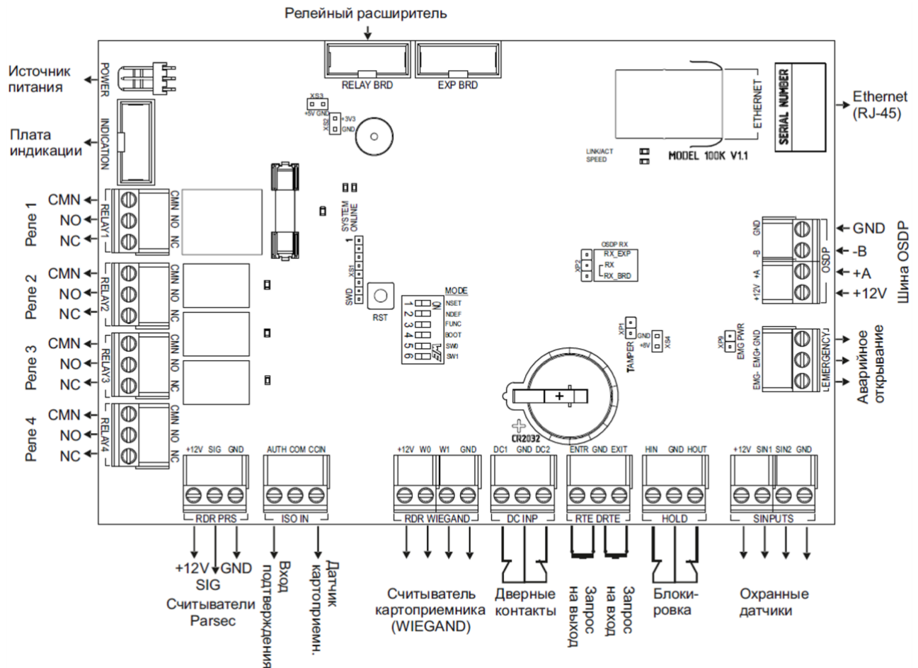
Рисунок 2. Схема платы контроллера ЛКД-КСТ-100000
