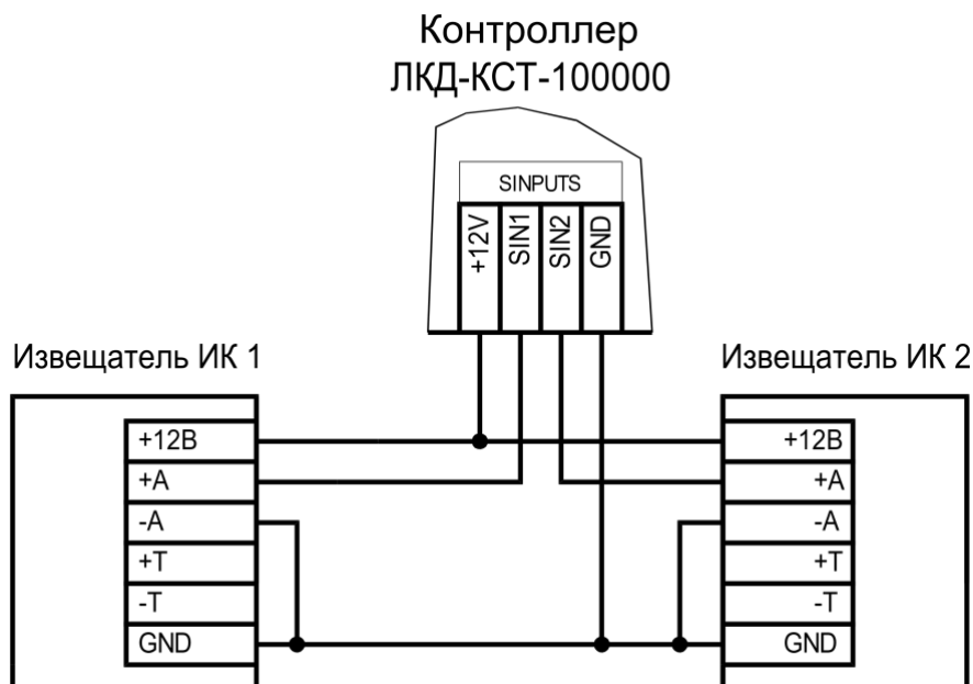
Рисунок 19. Схема подключения 2 охранных датчиков без контроля состояния линии
