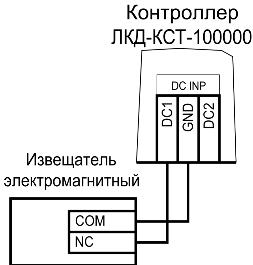
Рисунок 15. Схема подключения дверного контакта для точки прохода типа «дверь»
