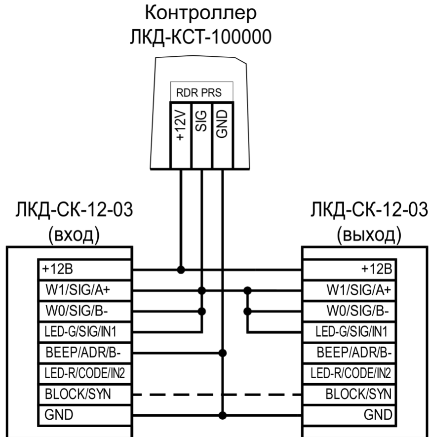
Рисунок 9. Схема подключения считывателей с интерфейсом ЛКД
