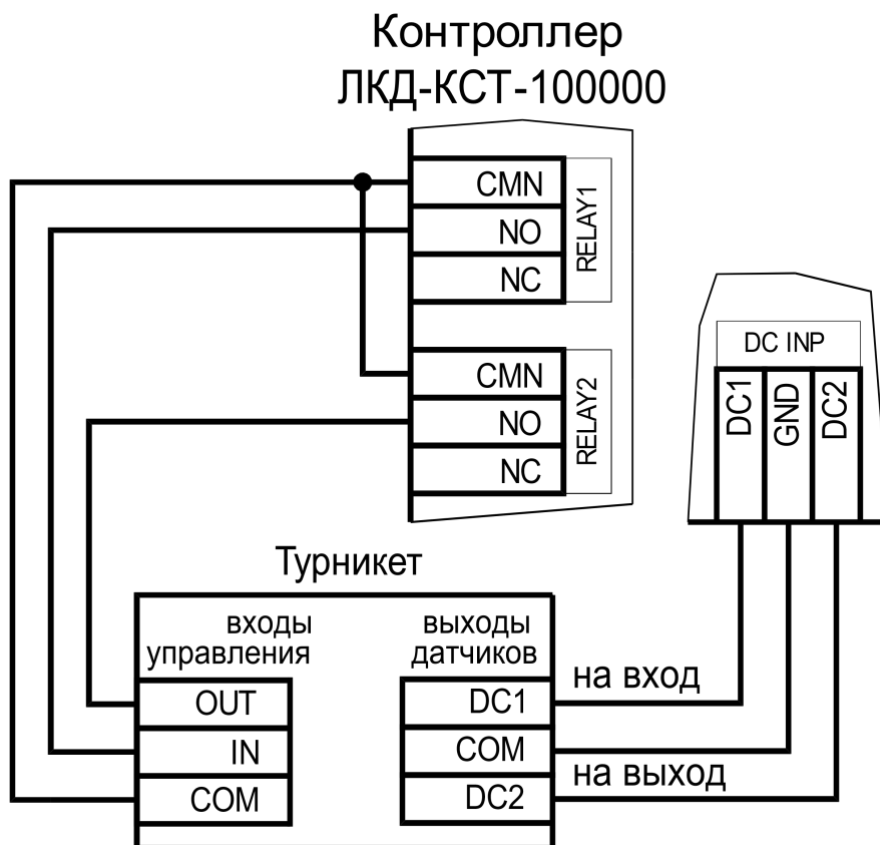
Рисунок 17. Схема подключения двух датчиков проворота турникета
