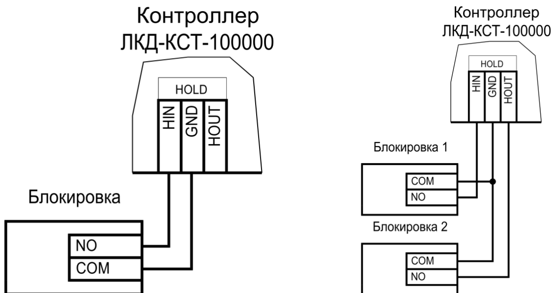
Рисунок 20. Схемы подключения блокировки контроллера
