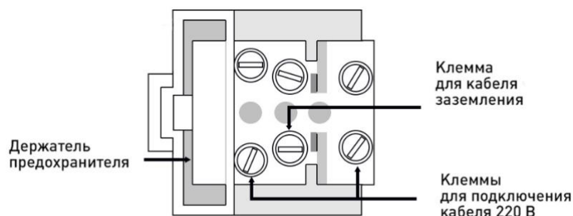
Рисунок 5. Клеммная колодка для кабеля питания
