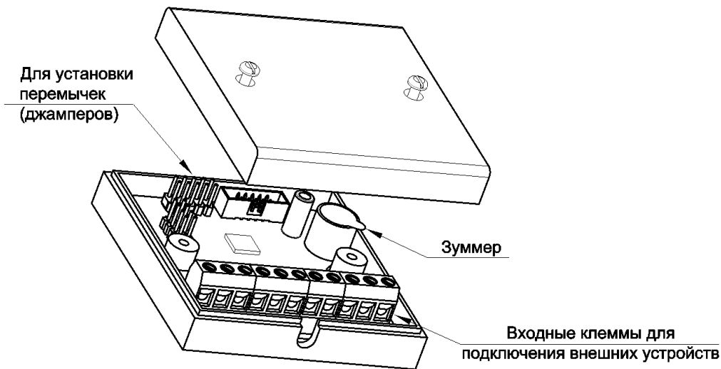
Рисунок 1 – Внешний вид и элементы подключения
