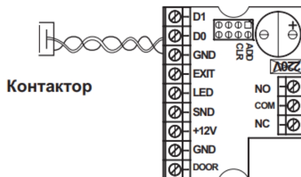
Рис.5 Подключение контактора.
