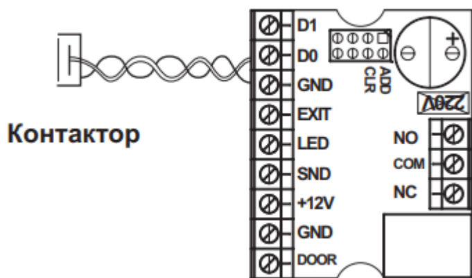
Рис.5 Подключение контактора.
