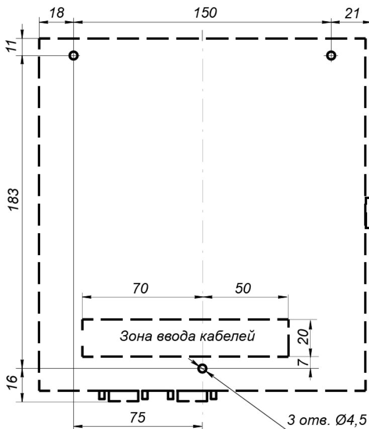
Рисунок 3. Разметка отверстий для монтажа контроллера
