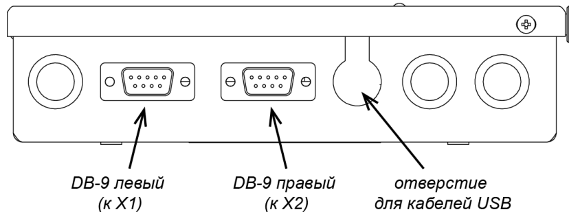
Рисунок 5. Расположение разъемов DB-9 (RS-232) на корпусе контроллера
