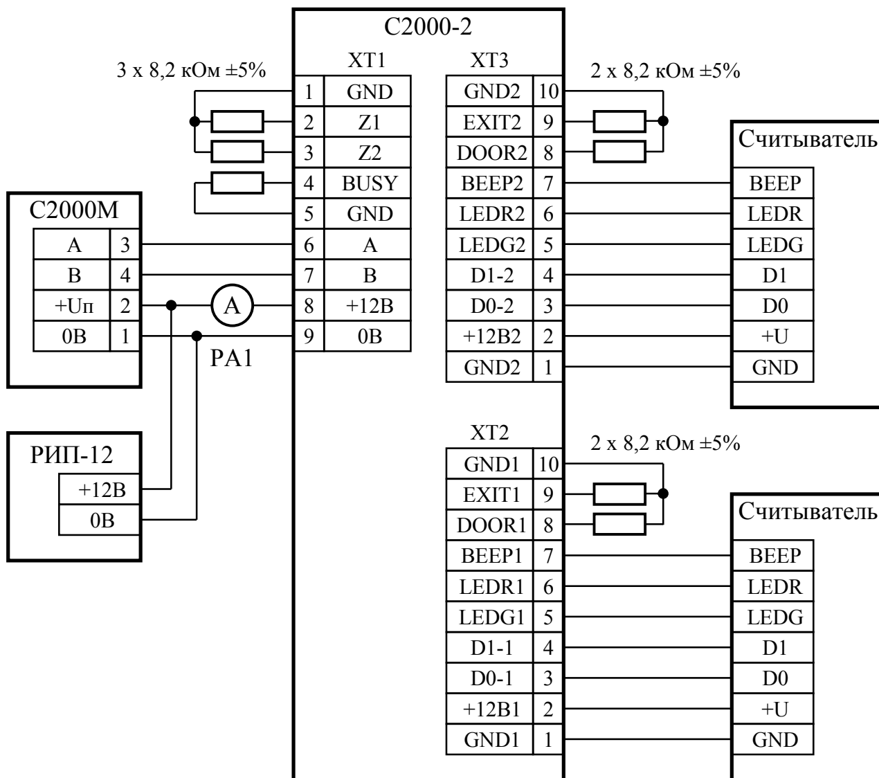
Рисунок 17 Схема подключения контроллера "C2000-2" при общей проверке
