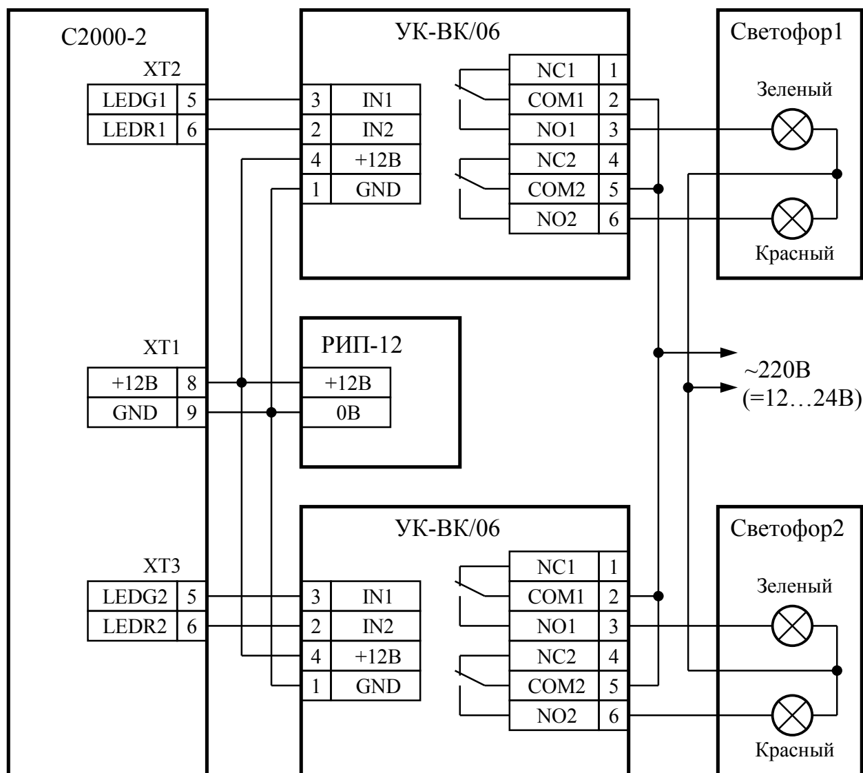
Рисунок 14 Схема подключения светофора к контроллеру "C2000-2" в режиме "Шлагбаум"
