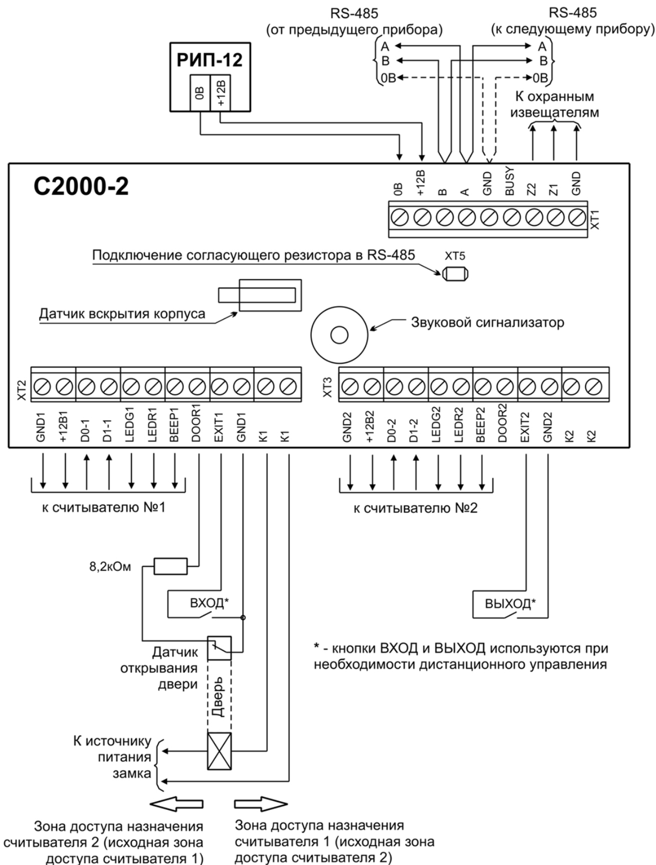
Рисунок 10 Схема подключения контроллера "C2000-2" в режиме "Одна дверь на вход/выход"
