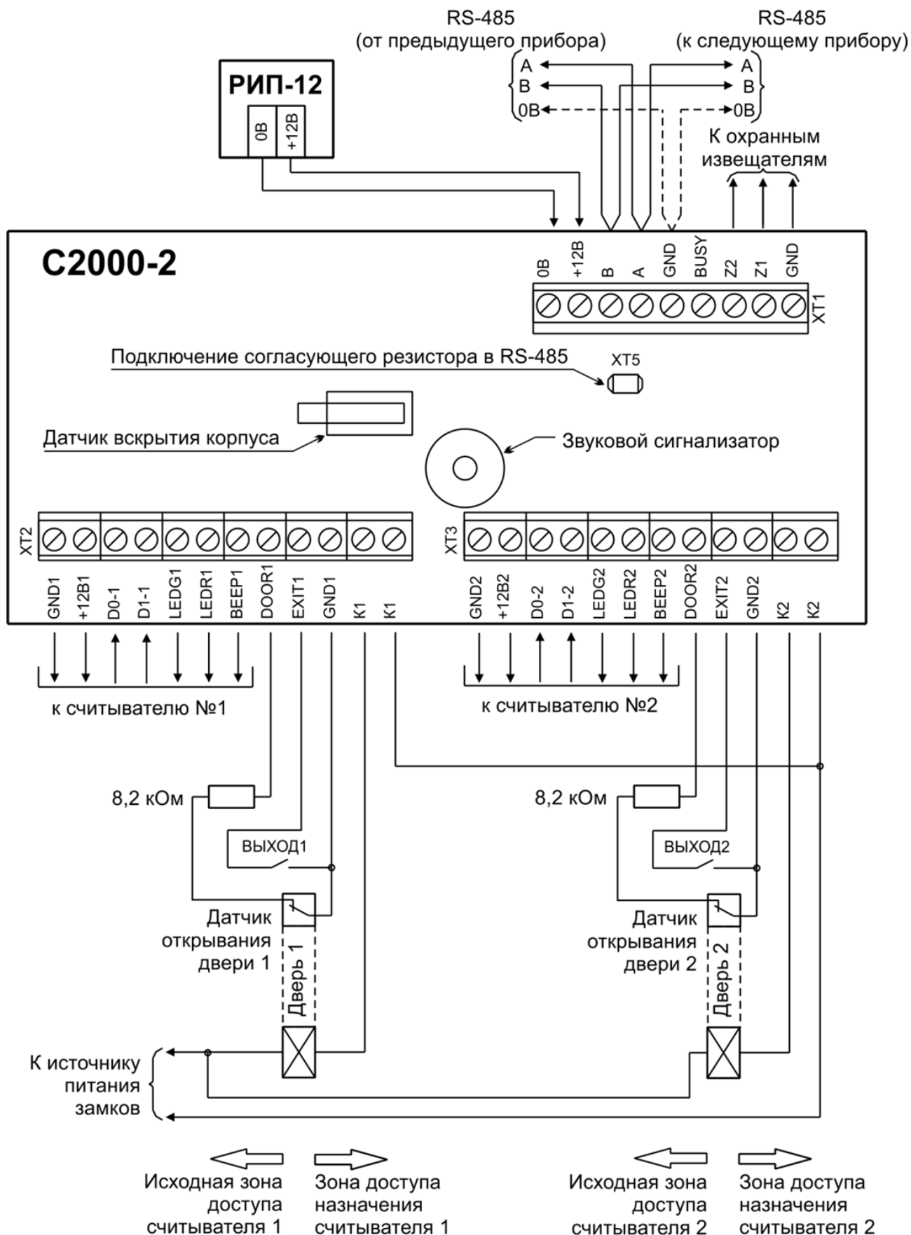
Рисунок 9 Схема подключения контроллера "C2000-2" в режиме "Две двери на вход"
