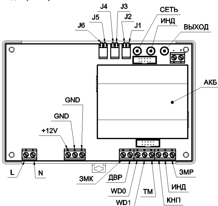
Рисунок 1 – Элементы подключения.
