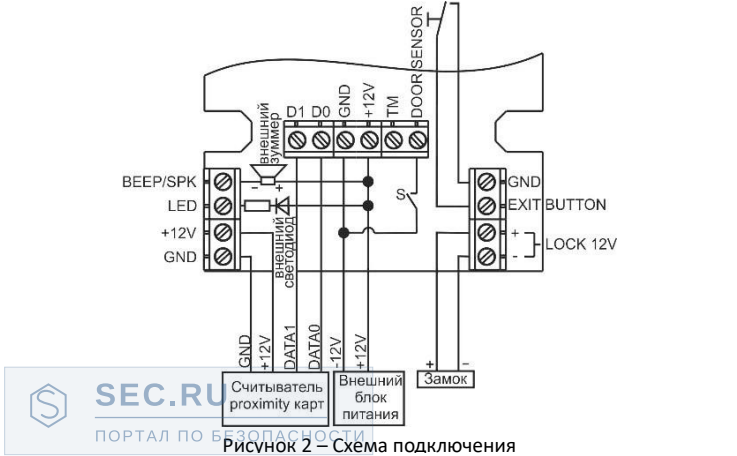
Рисунок 2 – Схема подключения
