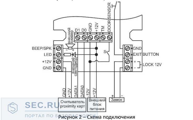
Рисунок 2 – Схема подключения
