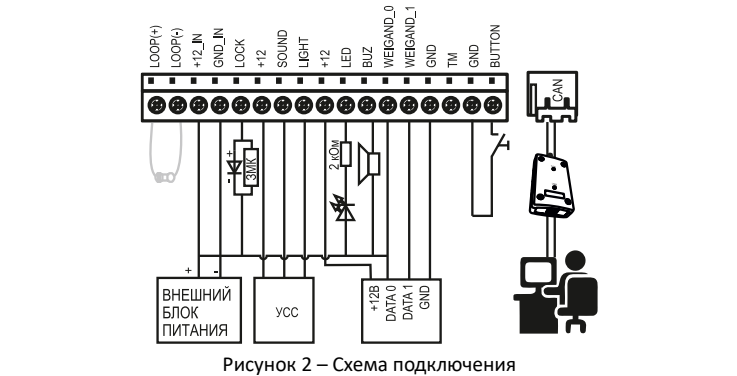
Рисунок 2 – Схема подключения
