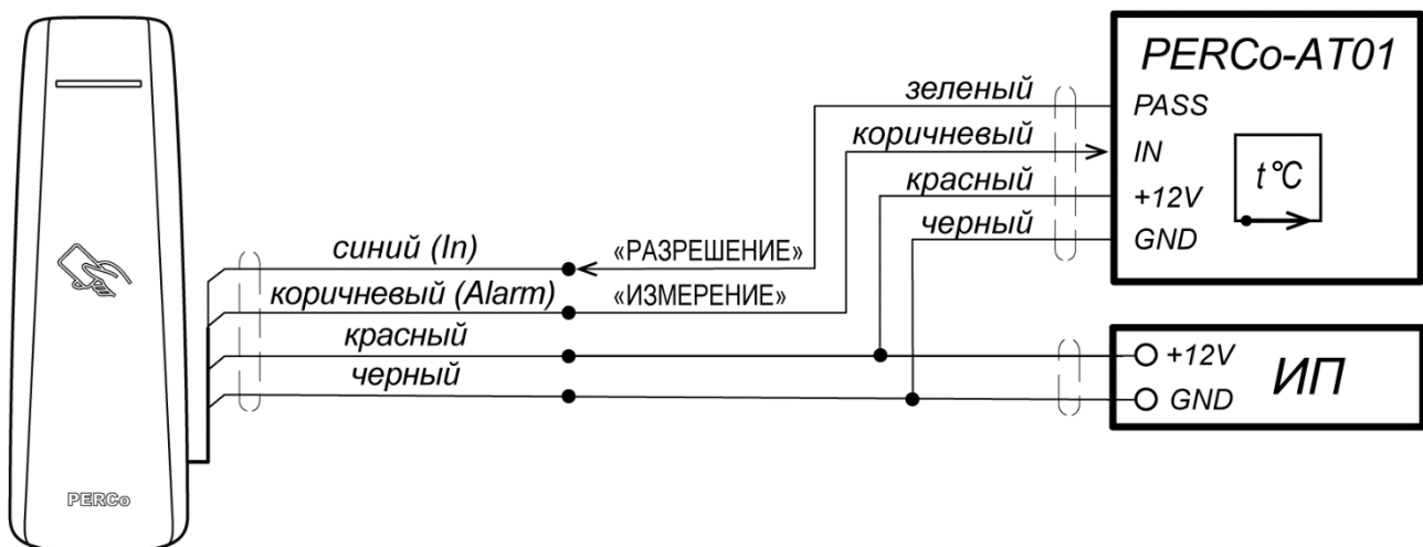
Рисунок 12. Схема подключения пирометра PERCo-AT01 к контроллеру CL15.7
