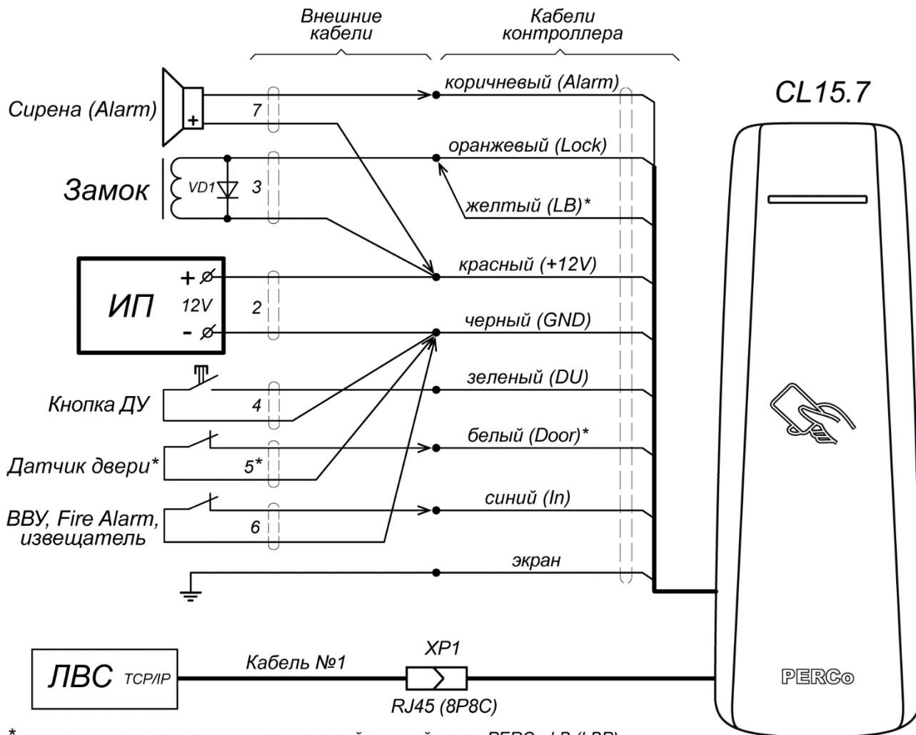
Рисунок 3. Схема подключений контроллера для управления односторонним замком
