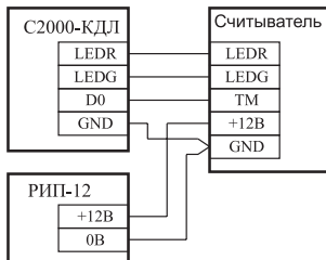
Рисунок 2 Схема подключения считывателей с интерфейсом Touch Memory
