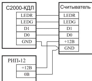
Рисунок 3 Схема подключения считывателей с интерфейсом Wiegand
