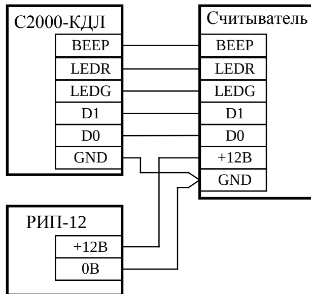
Рисунок 2.2.5 Схема подключения считывателей с интерфейсом Wiegand
