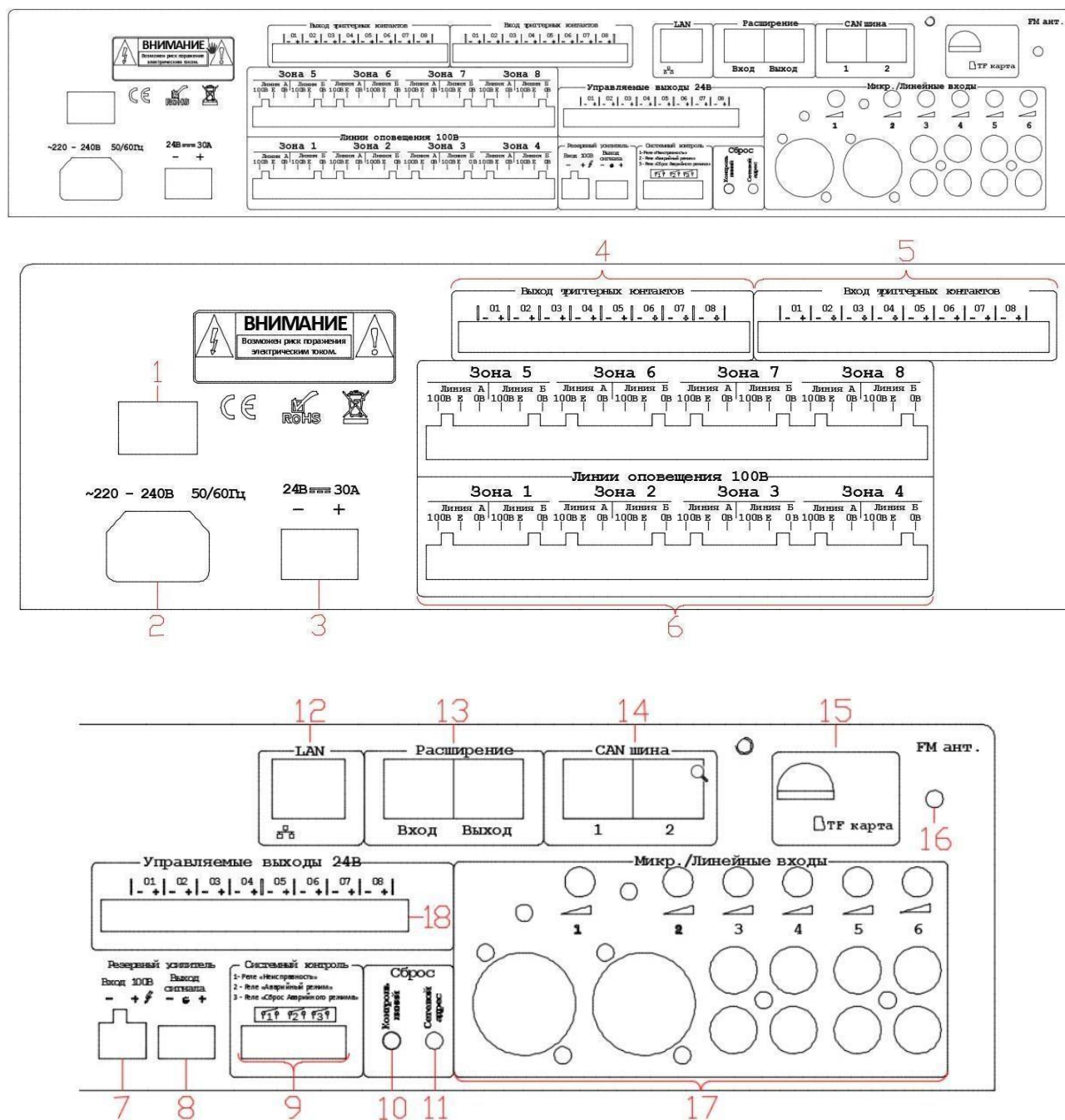
Рис. 2.1.3. Контроллер системы LPA-DUO-M (задняя панель)
